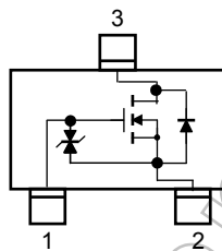
内部接続 (top view)
