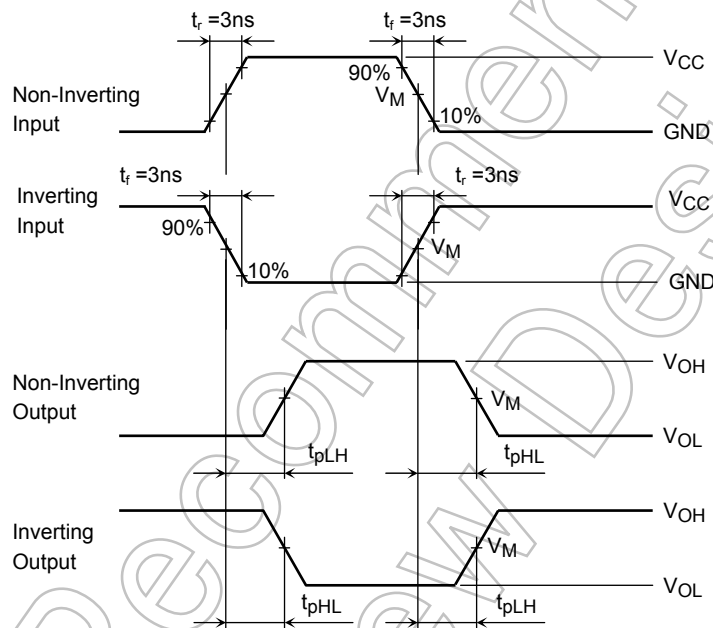
図 2 t_{pLH} , t_{pHL}
