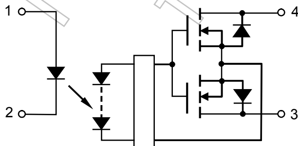
内部回路図
