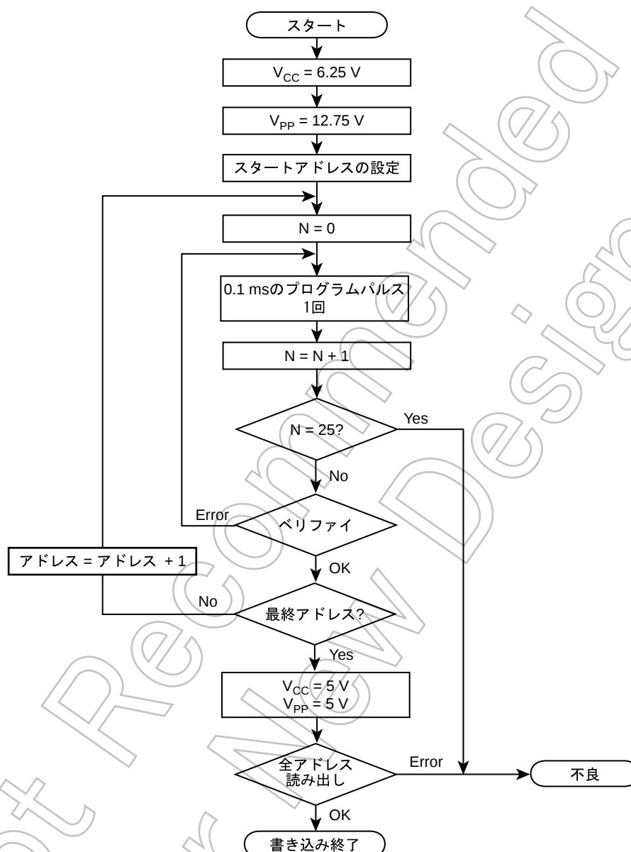
図 18-3 書き込みフローチャート
