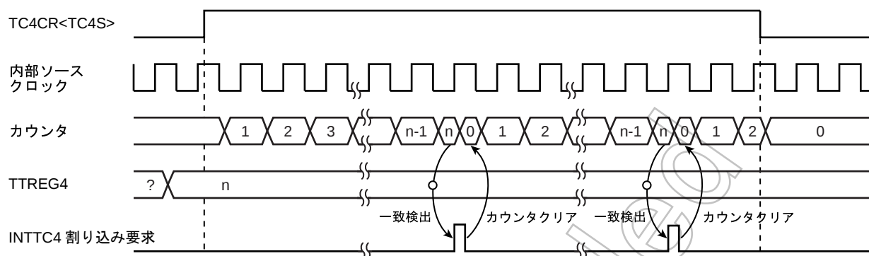
図 9-2 8ビットタイマモードタイミングチャート (TC4 の場合)
