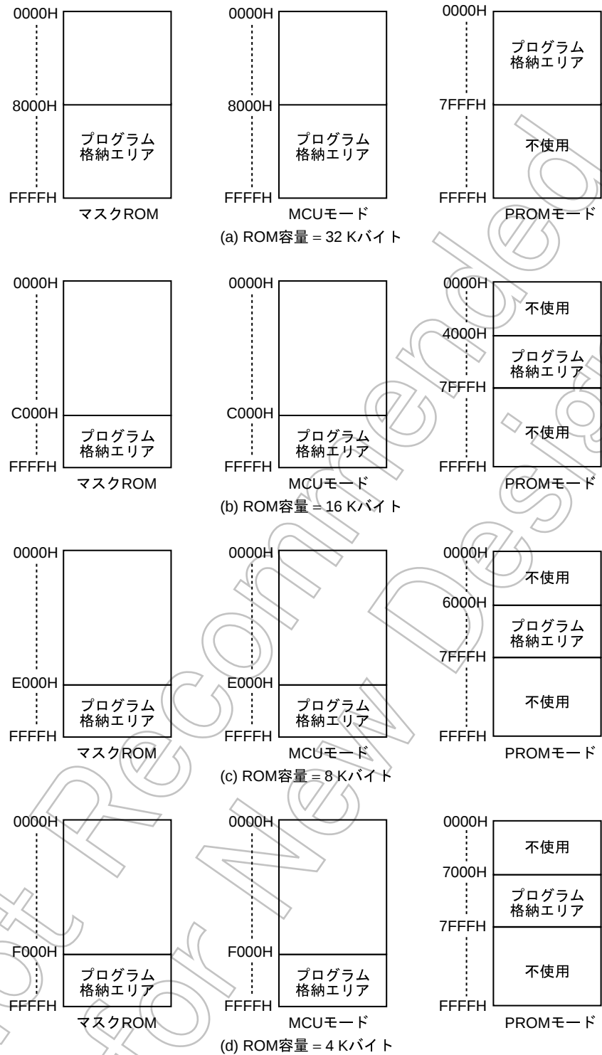
図 18-1 プログラム格納エリア
