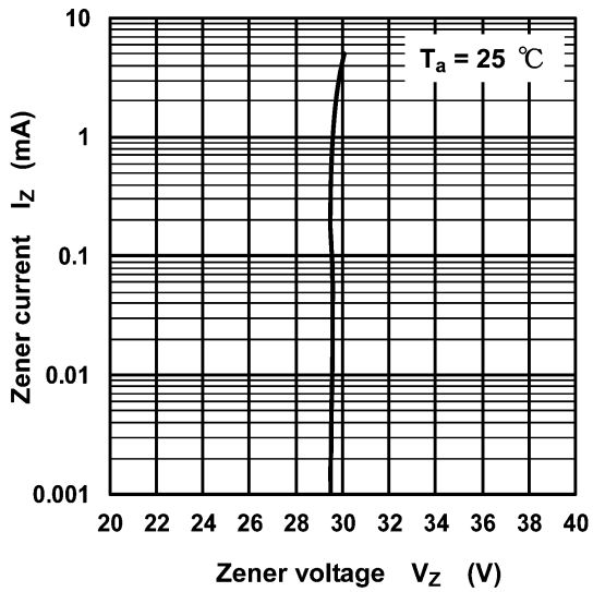
図 8.1 I_Z - V_Z
