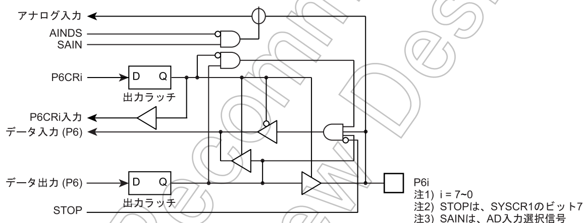
図 5-8 P6 ポート
