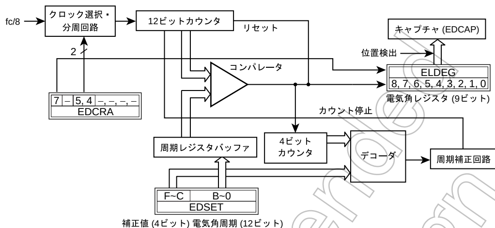
図 13-15 電気角タイマ回路
