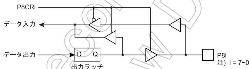
図 5-10 P8 ポート
