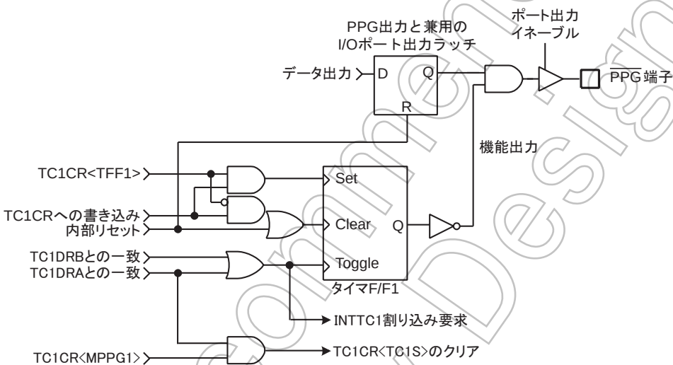
図 8-7 PPG 出力
