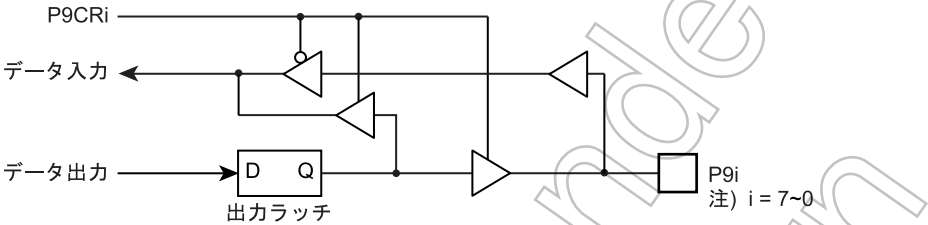
図 5-11 P9 ポート
