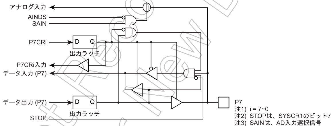
図 5-9 P7 ポート
