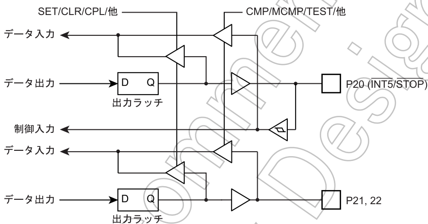
図 5-4 P2 ポート
