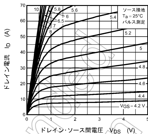
図 8.2 I_D - V_{DS}
