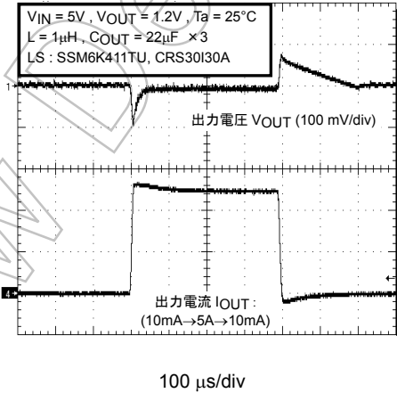
負荷応答特性
