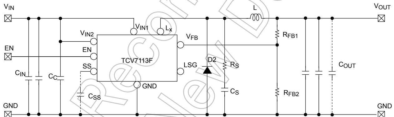
図 1 標準的な TCV7113F 応用回路例
