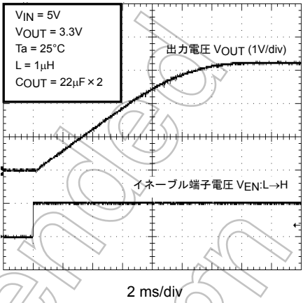
起動特性 ( C_{SS} = 0.1\mu F )
