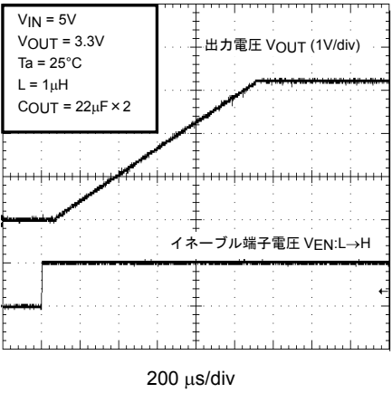
起動特性 (内部ソフトスタート時間)
