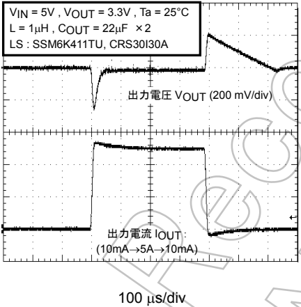
負荷応答特性
