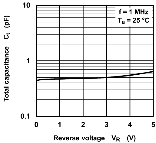
図 7.3 C_t - V_R
