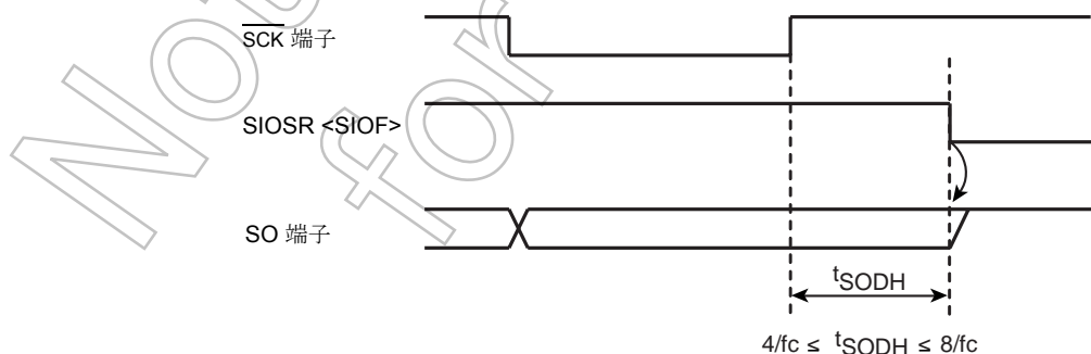
図 9-17 送受信終了時のデータ保持時間
