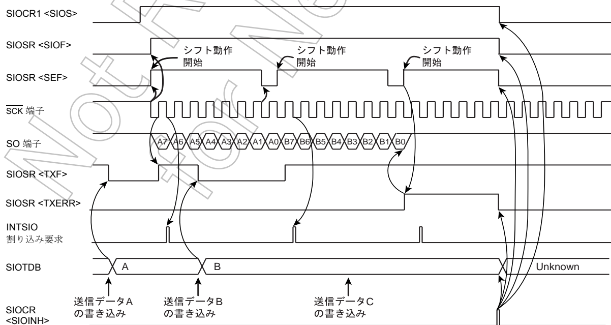
図 9-9 送信モードエラー処理の例
