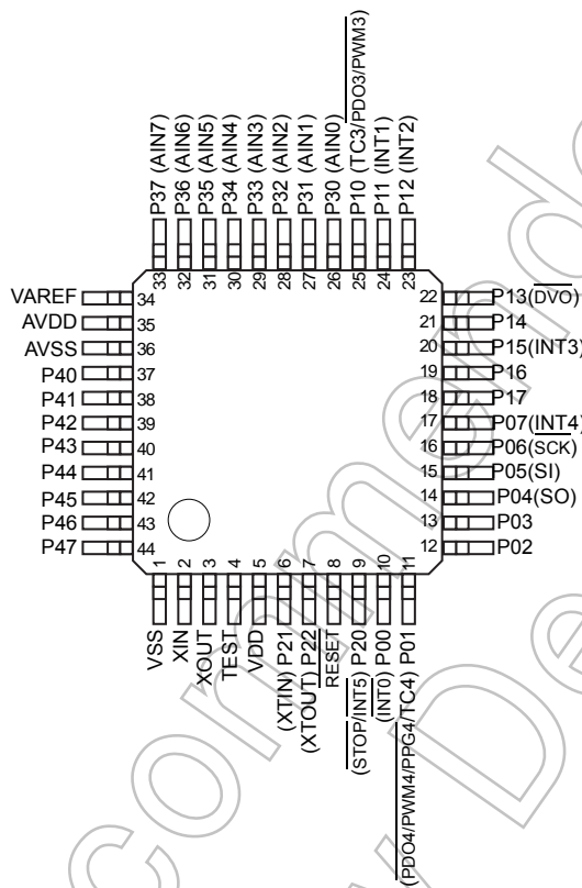
図 1-1 ピン配置図
