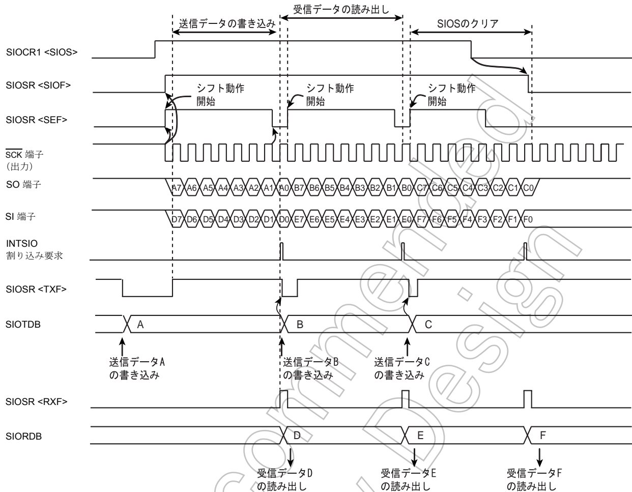
図 9-14 外部クロック、MSB 送受信の例
