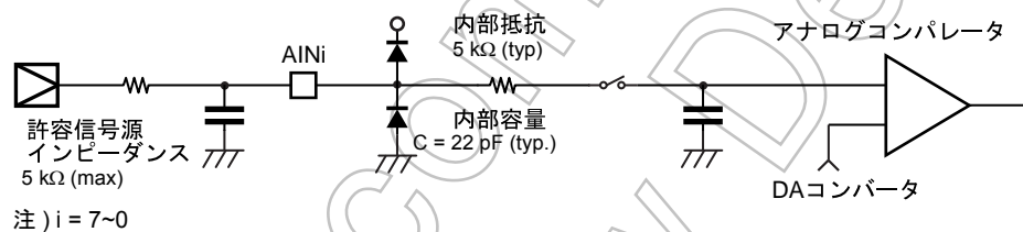
図 10-5 アナログ入力等価回路と入力端子処理例
