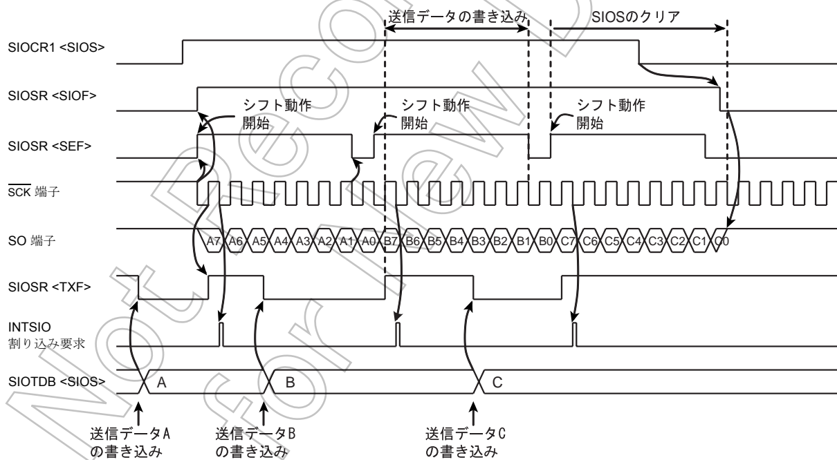
図 9-7 外部クロック、MSB 送信の例
