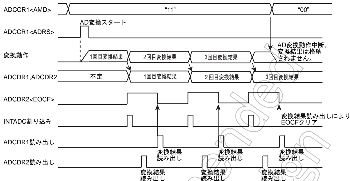
図 10-3 リピートモード
