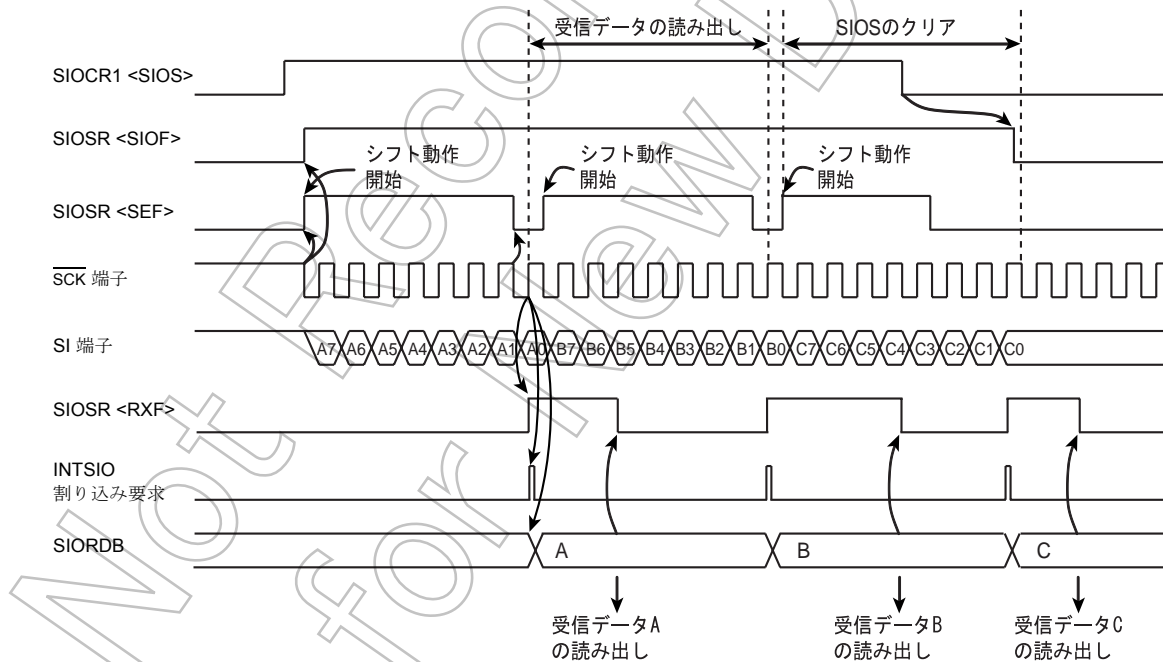
図 9-11 外部クロック、MSB 受信の例
