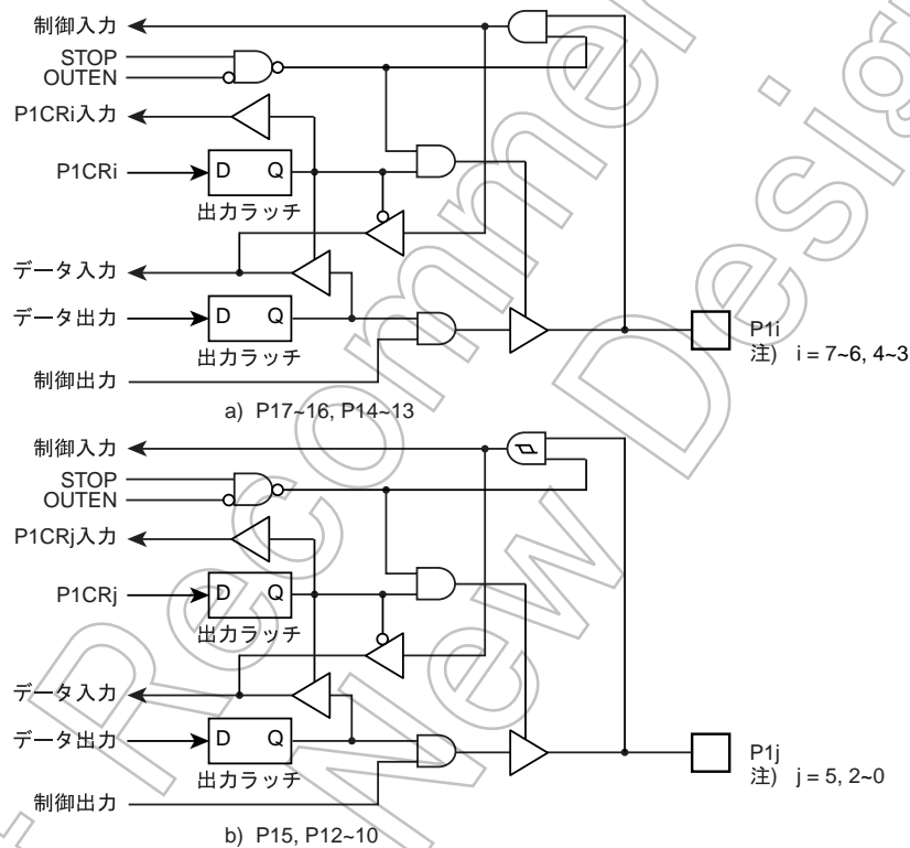
図 5-3 P1 ポート
