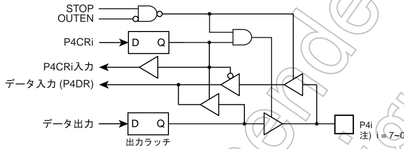
図 5-6 P4 ポート
