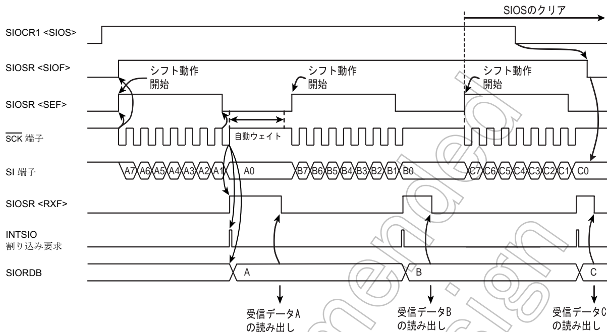
図 9-10 内部クロック、MSB 受信の例
