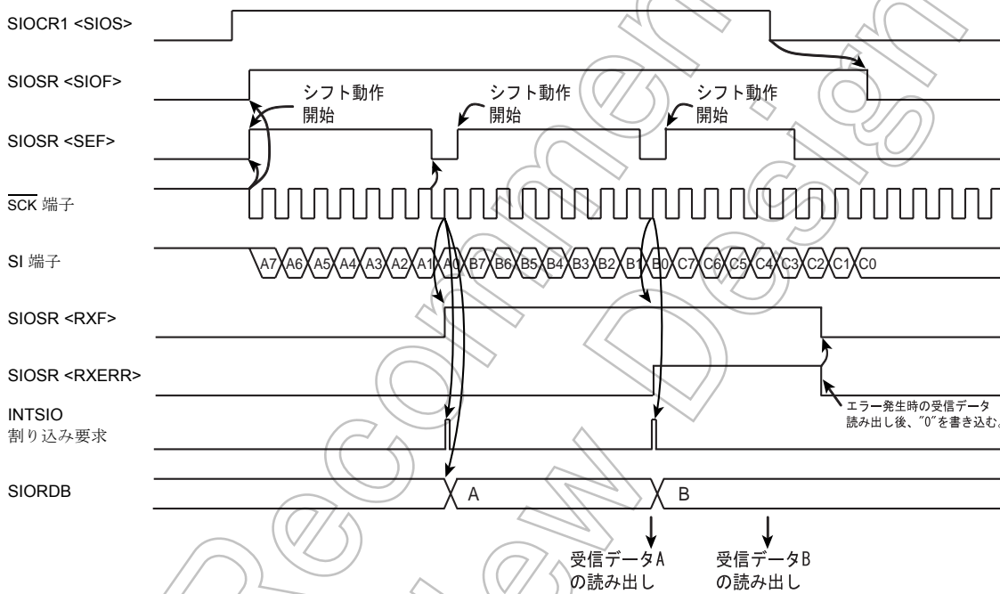
図 9-12 受信モードエラー処理の例
