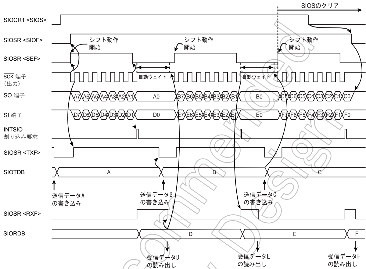
図 9-13 内部クロック、MSB 送受信の例
