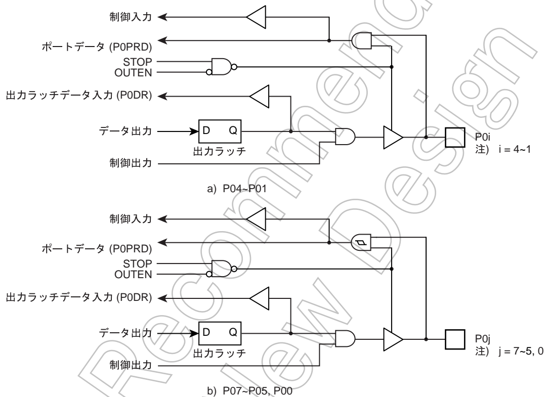
図 5-2 P0 ポート
