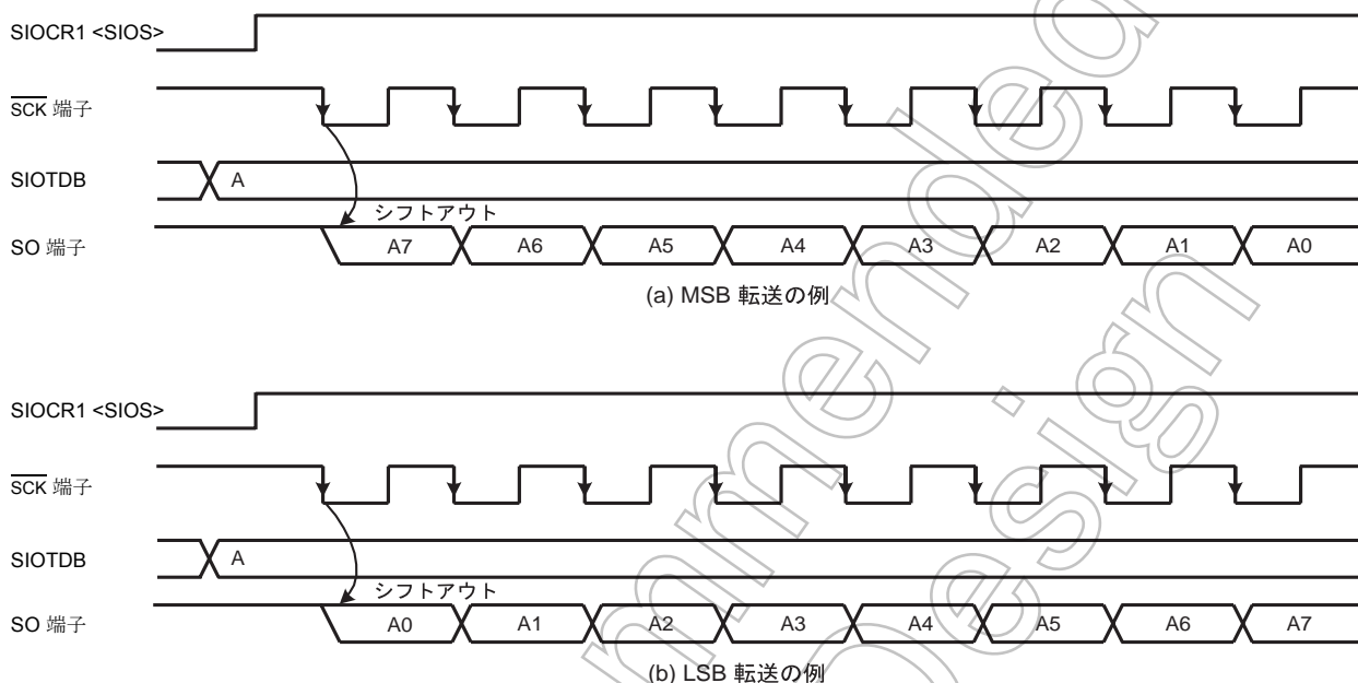
図 9-5 転送ビット方向 (送信モードの例)
