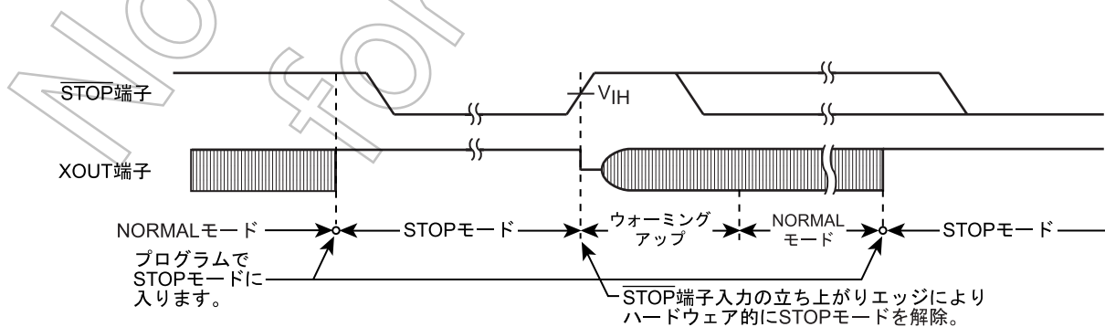
図 2-8 エッジ解除モード
