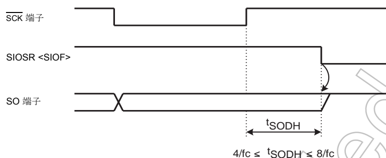
図 9-8 送信終了時のデータ保持時間
