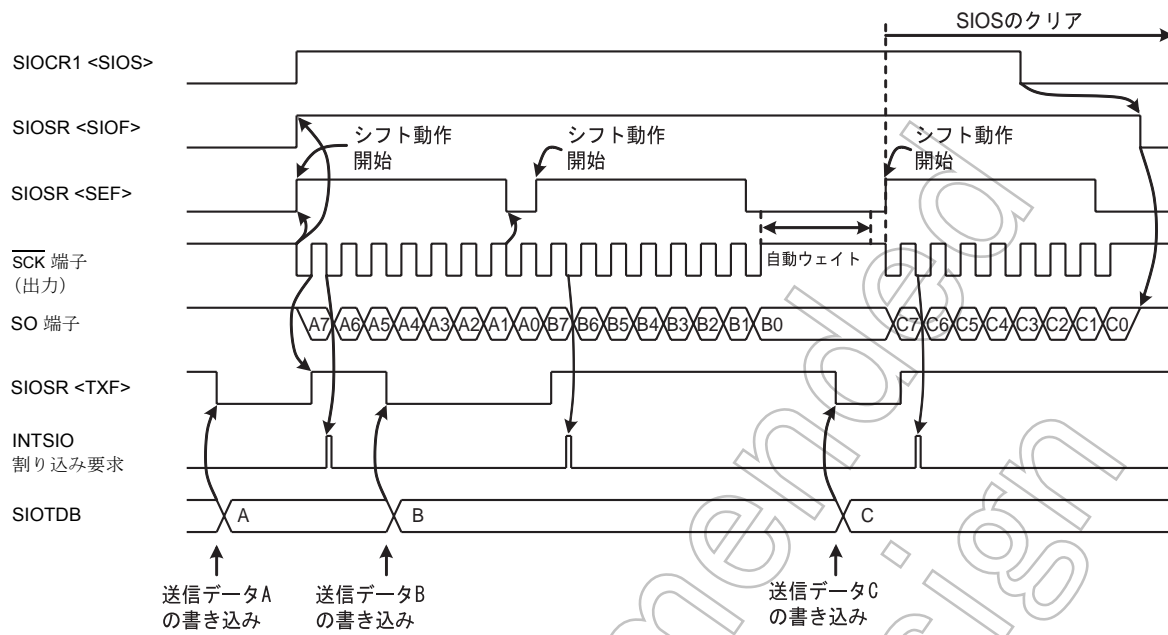
図 9-6 内部クロック、MSB 送信の例
