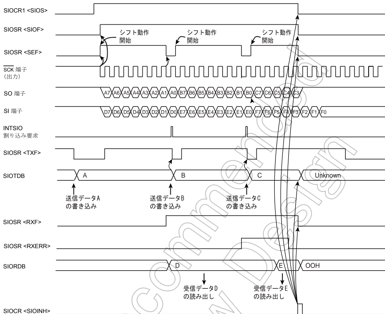
図 9-16 送受信モード ( 受信 ) エラー処理の例
