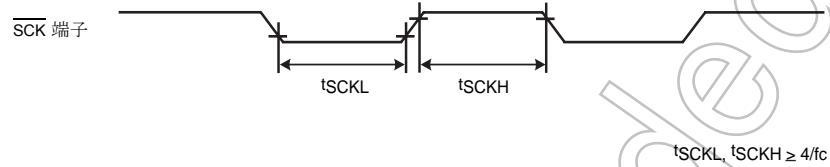
図 9-3 外部クロック
