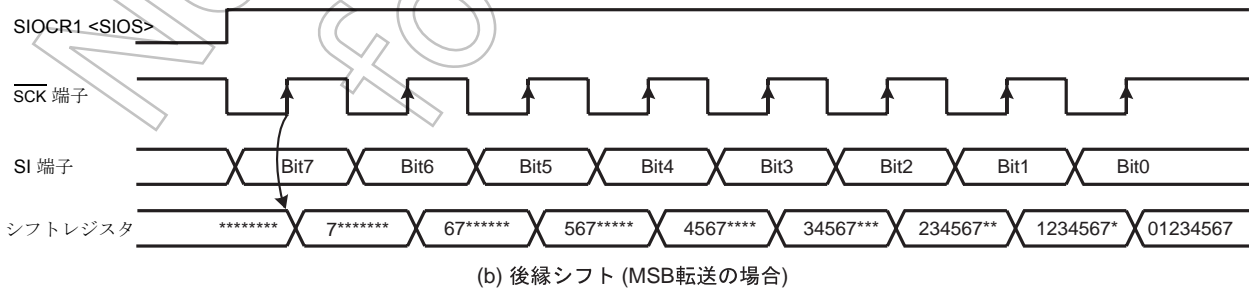
図 9-4 シフトエッジ
