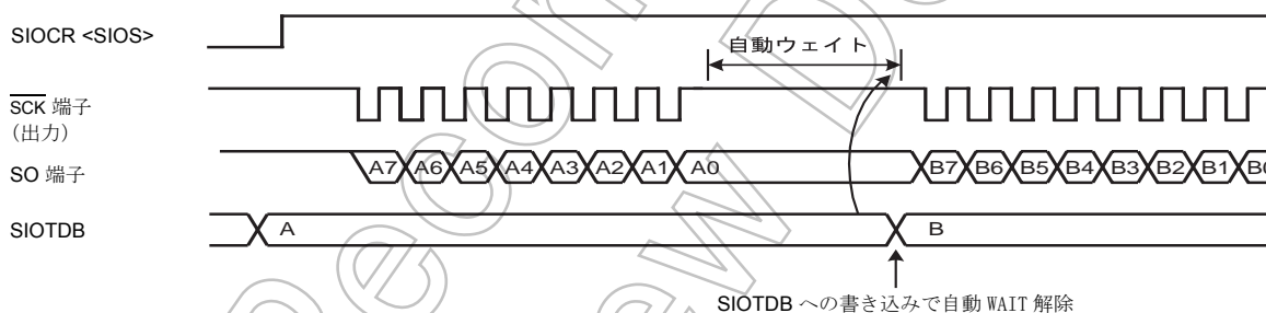
図 9-2 自動ウェイト機能 (送信モードの例)
