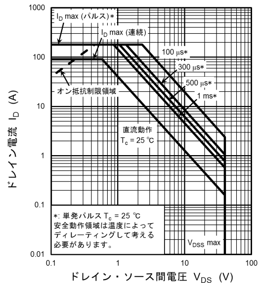
図 8.19 安全動作領域 (最大値 (保証値))
