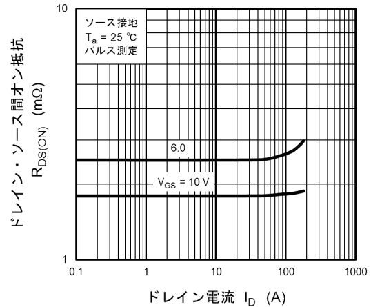
図 8.8 R_{DS(ON)} - I_D
