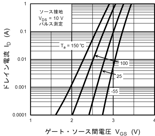
図 8.7 I_D - V_{GS}
