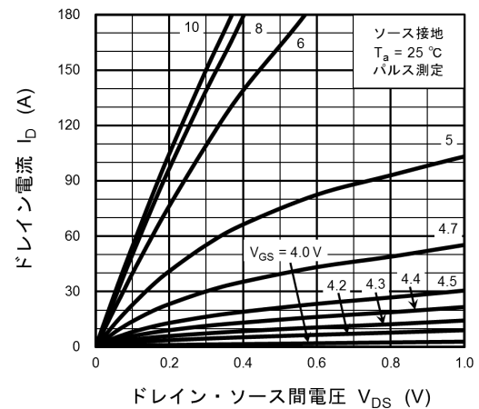
図 8.2 I_D - V_{DS}
