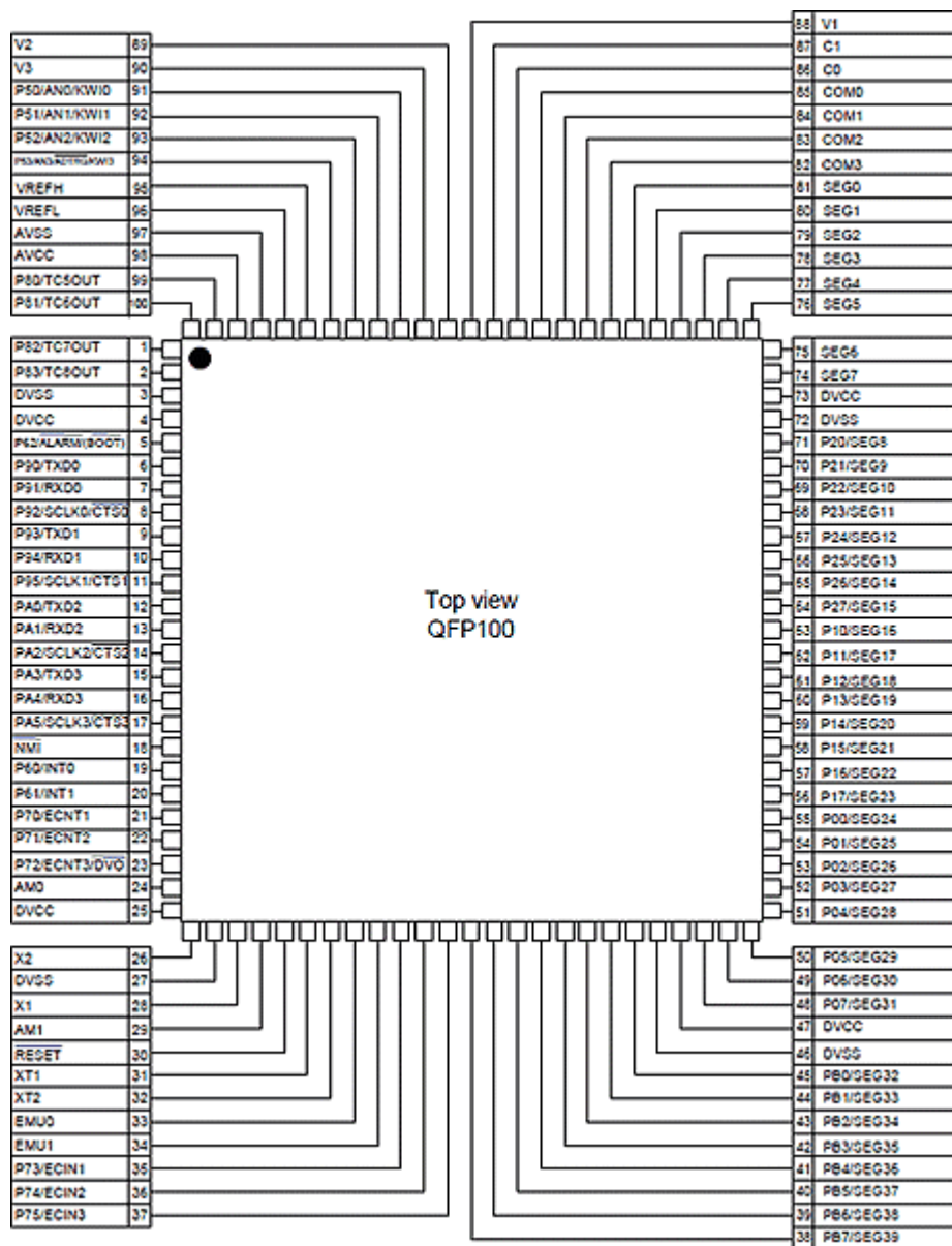
パッケージ名称 LQFP100-P-1414-0.50F
