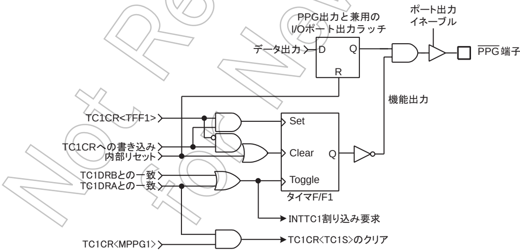
図 8-7 PPG 出力
