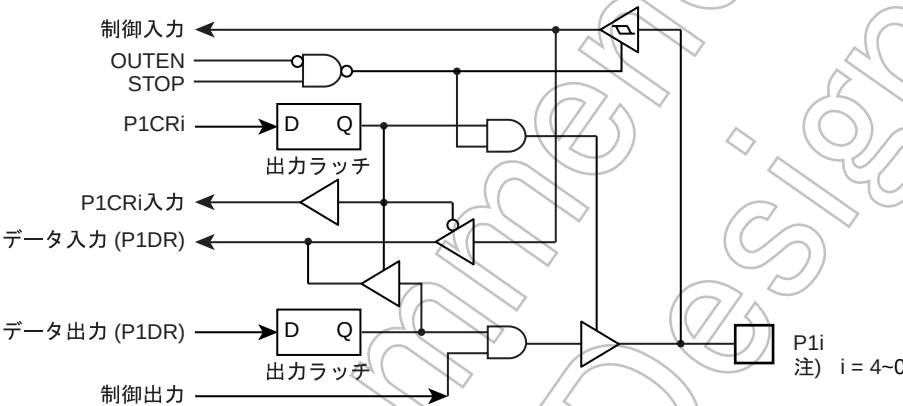
図 5-3 P1 ポート
