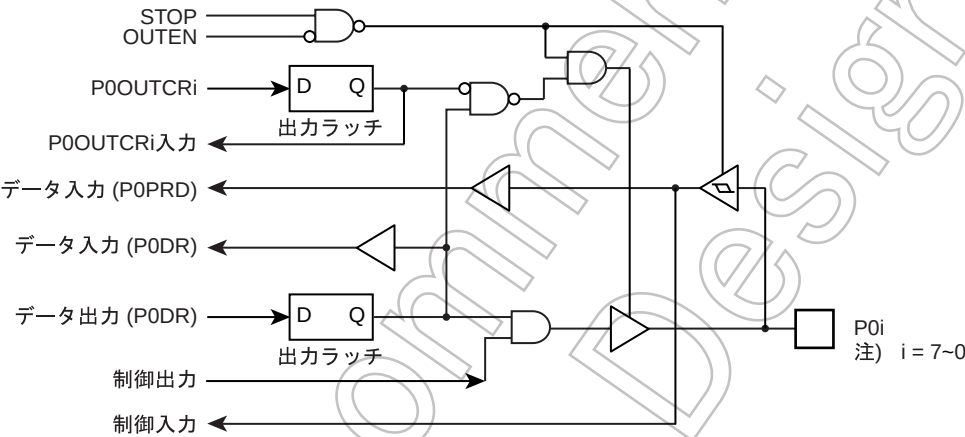
図 5-2 P0 ポート
