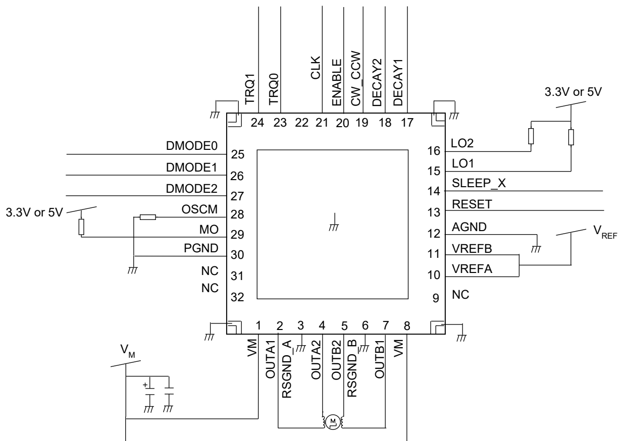
図 10.1 応用回路例
