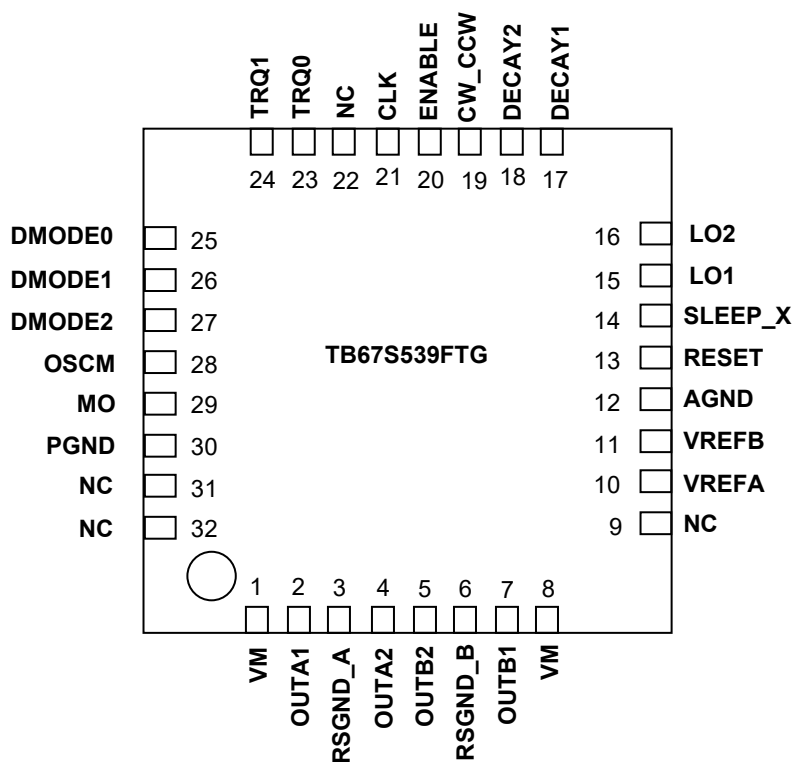
图 4.4.1 端子配置图
