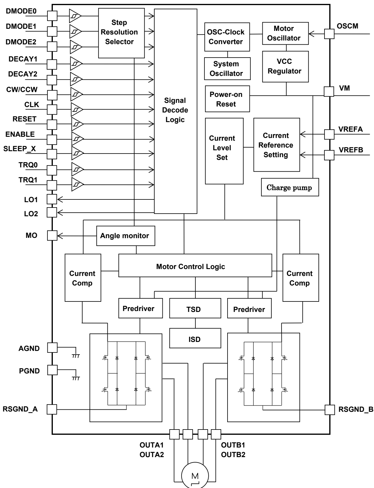
図 3.3.1 ブロック図
