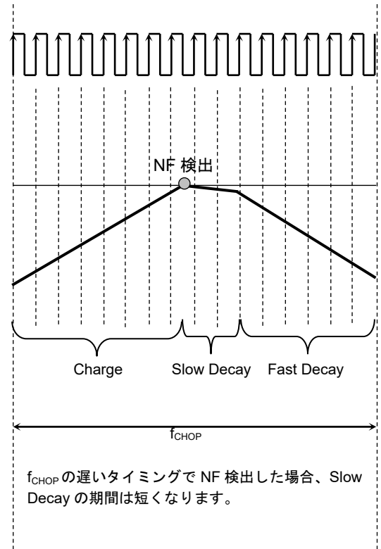
図 6.11 定電流 PWM 動作の各時間 (2)
