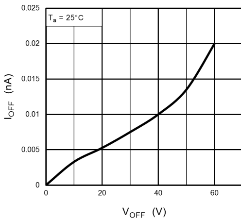
Fig. 12.9 I_{OFF} - V_{OFF}
