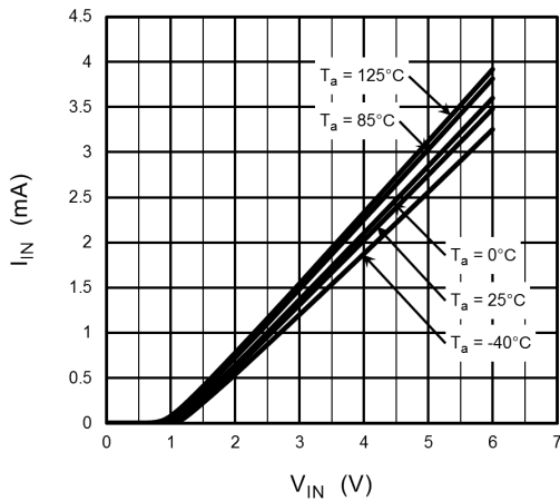
Fig. 12.1 I_{IN} - V_{IN}
