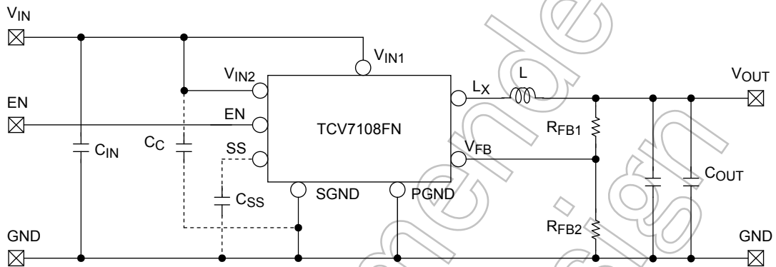
図 1 TCV7108FN 応用回路例
