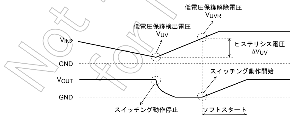
図4 低電圧保護動作
