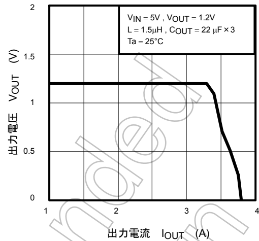
過電流特性
