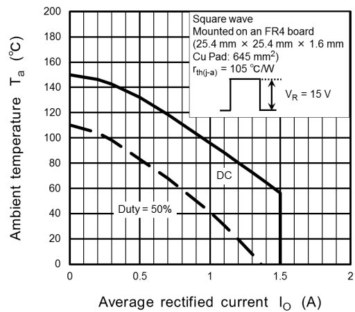
Fig. 9.6 T_a - I_O
