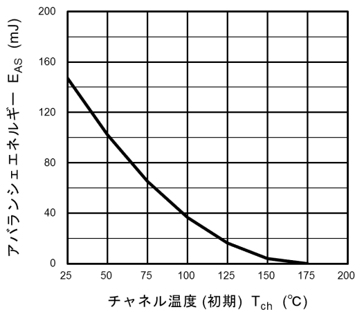
チャンネル温度 (初期) T_{ch} ( ^\circ\text{C} ) 図 8.15 E_{AS} - T_{ch} (最大値 (保証値))
