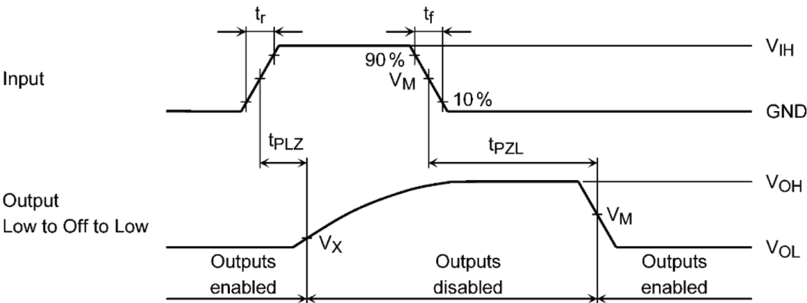
图 9.8.1 tPLZ, tPZL
