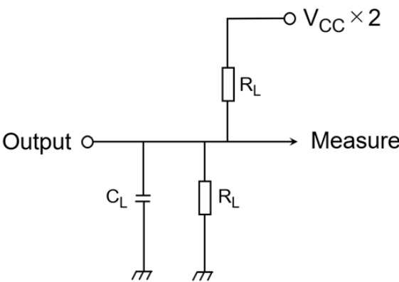
图 9.7.1 AC電氣的特性測定回路
