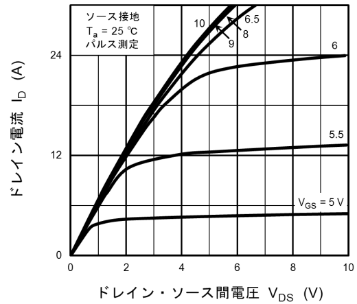
図 8.2 I_D - V_{DS}
