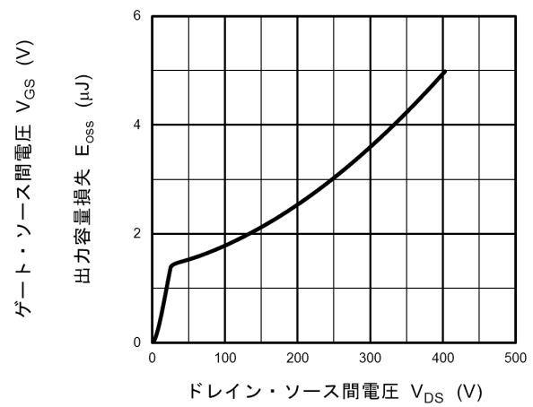
図 8.12 E_{oss} - V_{DS}
