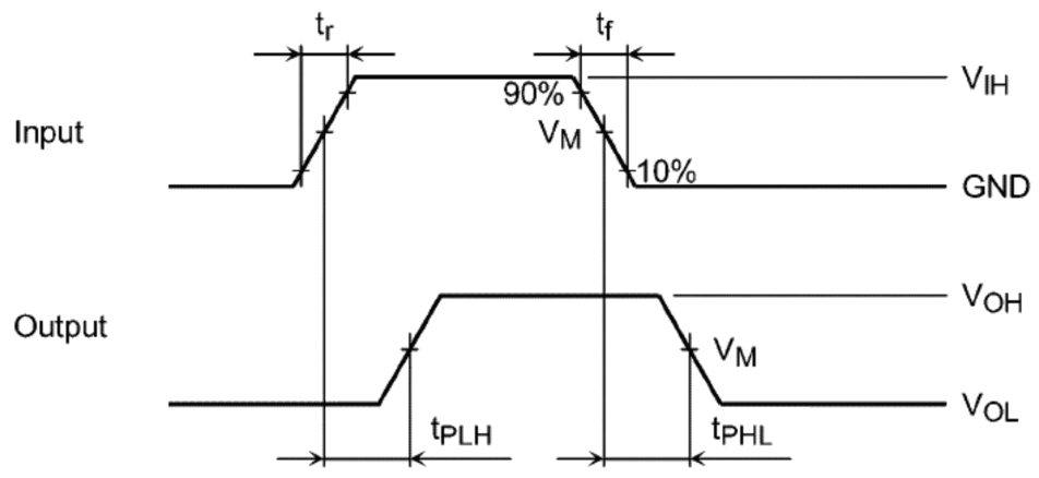
図 11.6.1 tPLH, tPHL
