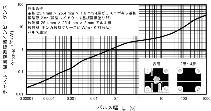
図 8.18 Z_{th(ch-a)} - t_w (参考値)
