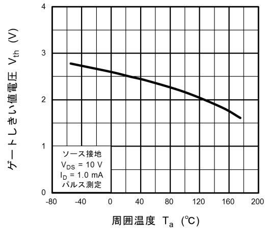
図 8.8 V_{th} - T_a
