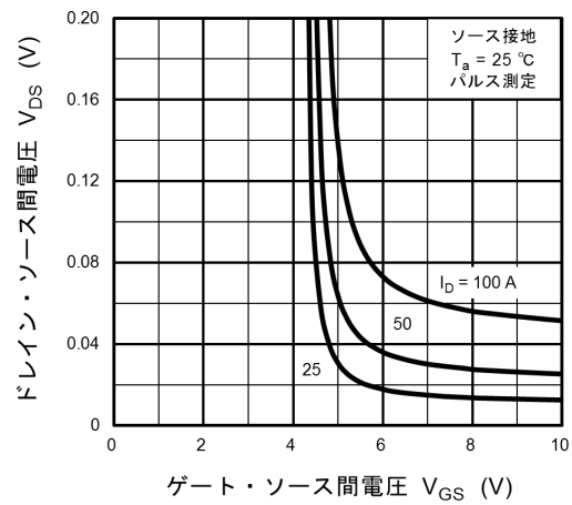
図 8.4 V_{DS} - V_{GS}
