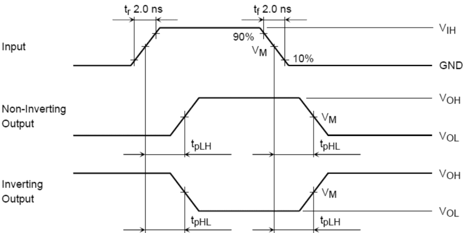
図 12.6.1 t_{pLH} , t_{pHL}
