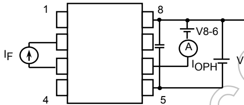
図 1 I_{OPH} 測定回路図
