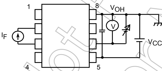
図 3 V_{OH} 測定回路図
