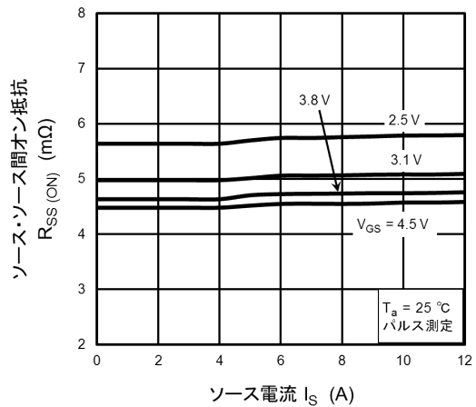
図 9.2 R_{SS(ON)} - I_S
