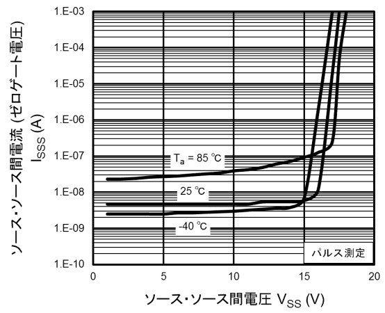
図 9.6 I_{CSS} - V_{SS}
