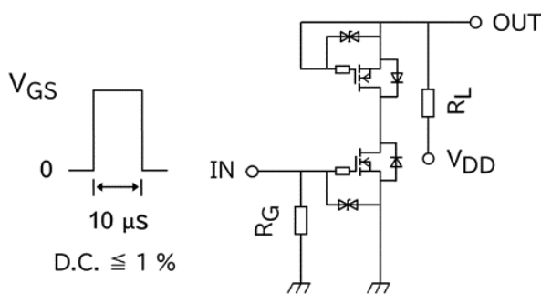
図 6.3.1 スイッチング時間の測定回路
