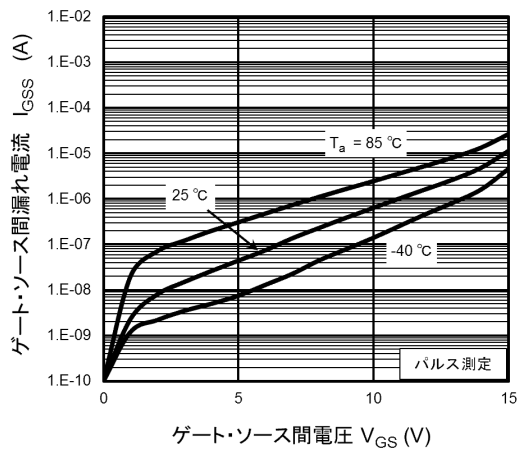
図 9.5 I_{GSS} - V_{GS}
