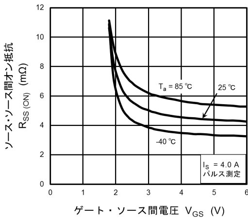
図 9.3 R_{SS(ON)} - V_{GS}
