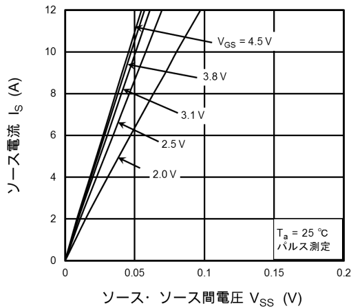
図 9.1 I_S - V_{SS}
