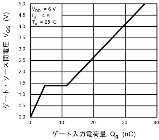
図 9.7 ダイナミック入力特性
