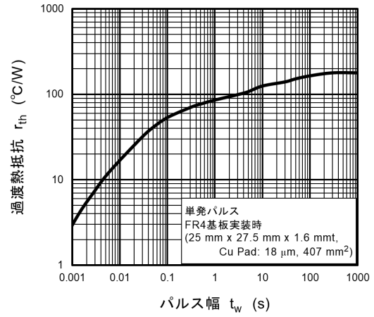
図 9.8 r_{th} - t_w
