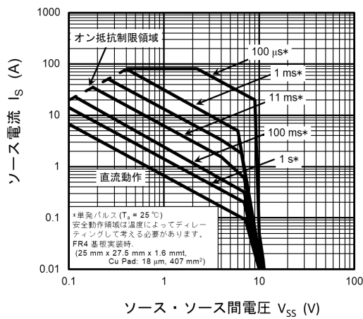
図 9.9 安全動作領域
