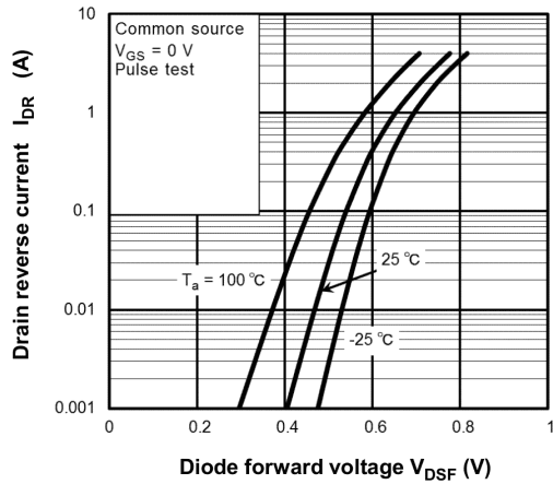
Fig. 9.7 I_{DR} - V_{DSF}
