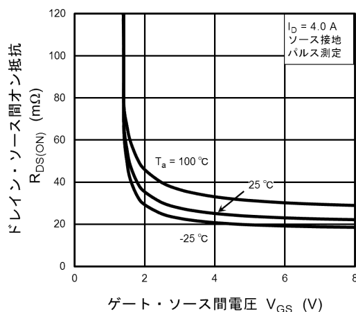
図 9.3 R_{DS(ON)} - V_{GS}
