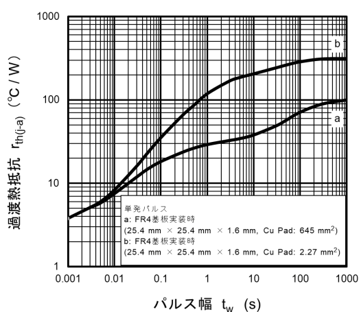
図 9.11 r_{th(j-a)} - t_w
