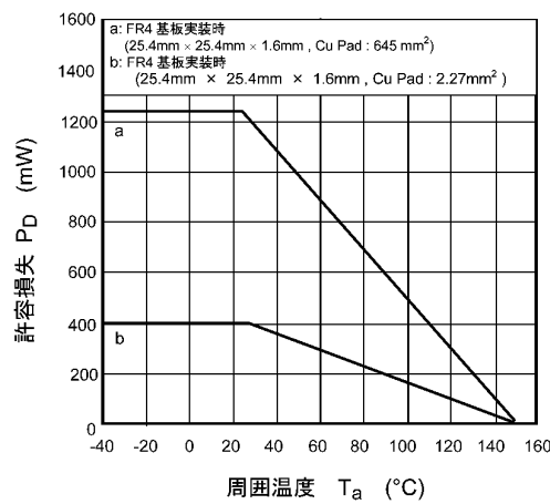
図 9.13 P_D - T_a
