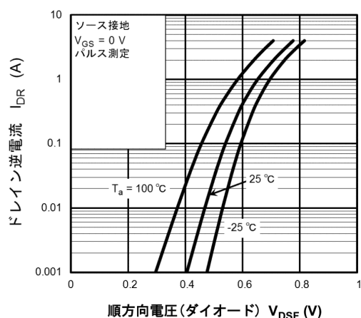
図 9.7 I_{DR} - V_{DSF}
