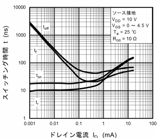
図 9.9 t - I_D
