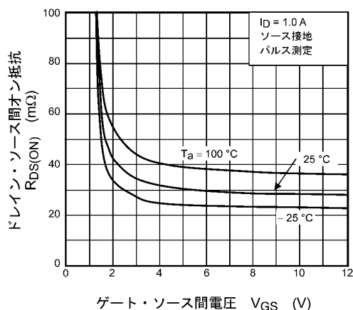
図 9.3 R_{DS(ON)} - V_{GS}
