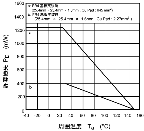
図 9.15 P_D - T_a
