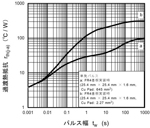
図 9.13 r_{th(j-a)} - t_w
