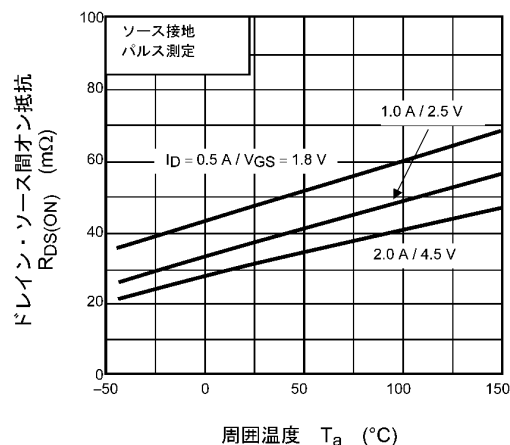
図 9.6 R_{DS(ON)} - T_a
