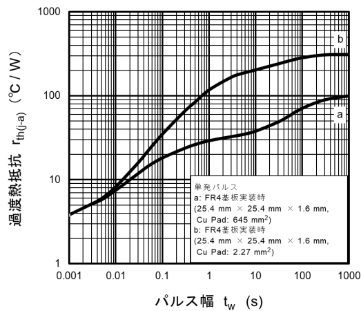
図 9.13 r_{th(j-a)} - t_w
