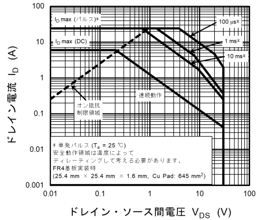
図 9.14 安全動作領域
