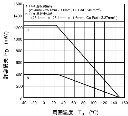
図 9.15 P_D - T_a
