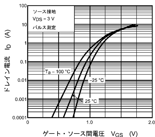
図 9.2 I_D - V_{GS}
