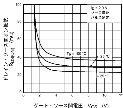
図 9.4 R_{DS(ON)} - V_{GS}
