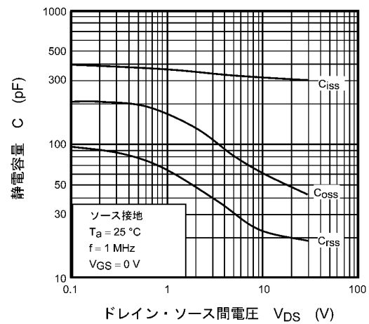
図 9.10 C - V_{DS}
