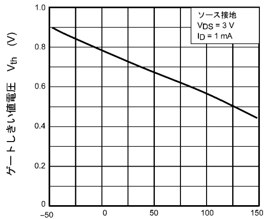
図 9.7 V_{th} - T_a
