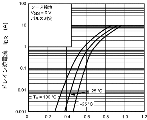
図 9.9 I_{DR} - V_{DSF}
