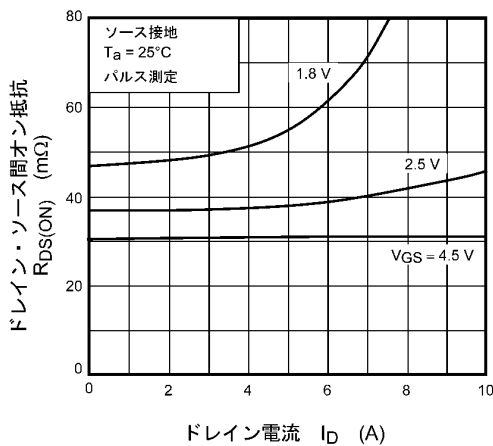
図 9.5 R_{DS(ON)} - I_D
