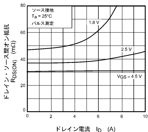
図 9.5 R_{DS(ON)} - I_D
