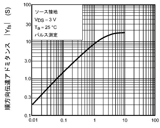
図 9.8 |Y_{fs}| - I_D
