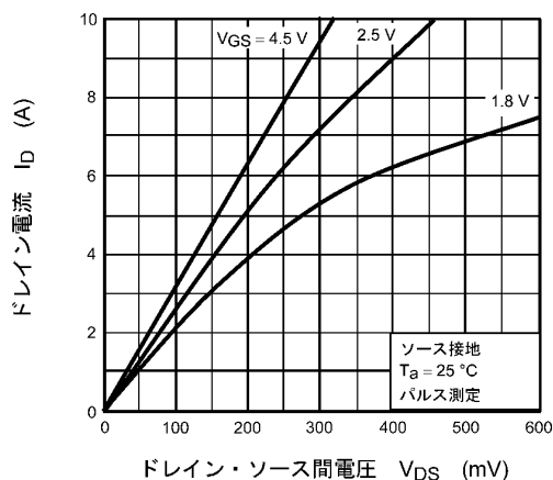
図 9.1 I_D - V_{DS}
