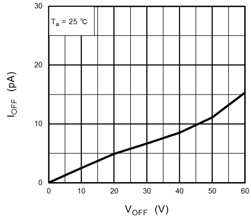
Fig. 12.8 I_{OFF} - V_{OFF}
