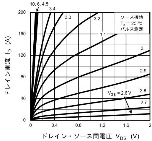
図 8.2 I_D - V_{DS}
