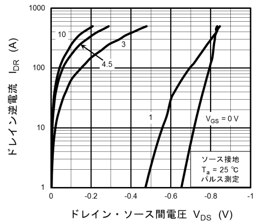
図 8.6 I_{DR} - V_{DS}
