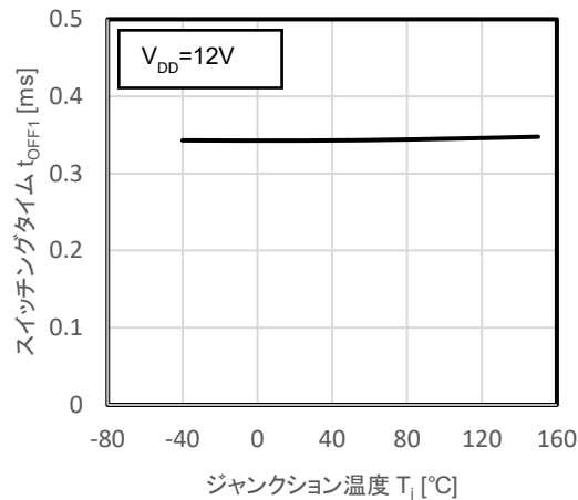
図 12.36 t_{OFF1} - T_j
