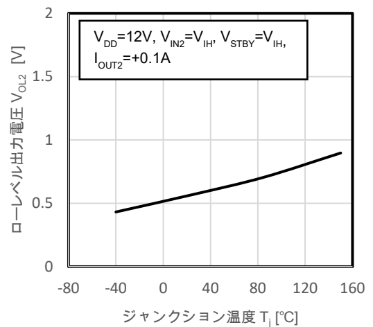
図 12.18 V_{OL2} - T_j
