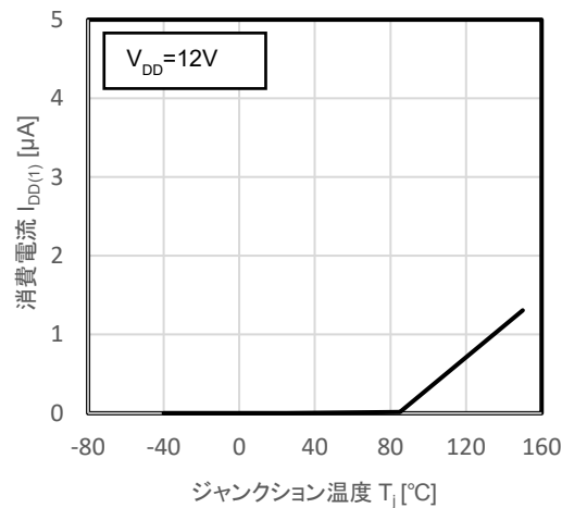
図 12.1 I_{DD(1)} - T_j
