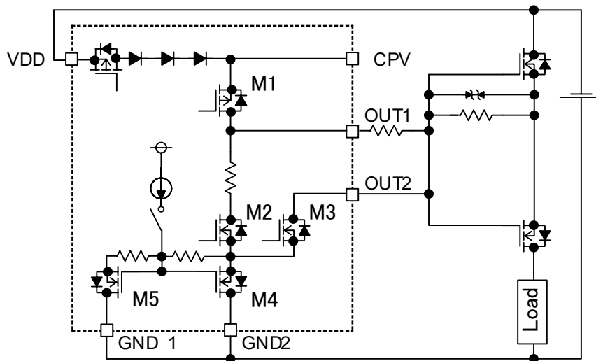
図 7.3 電源逆接保護
