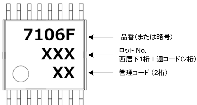
図 13.2 現品表示
