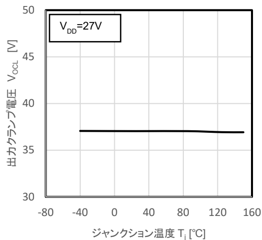
図 12.14 V_{OCL} - T_j
