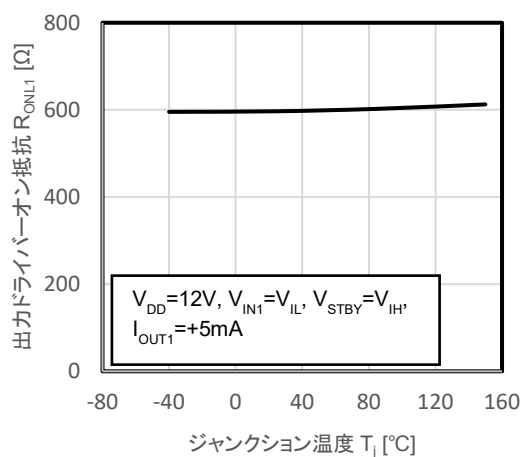
図 12.32 R_{ONL1} - T_j
