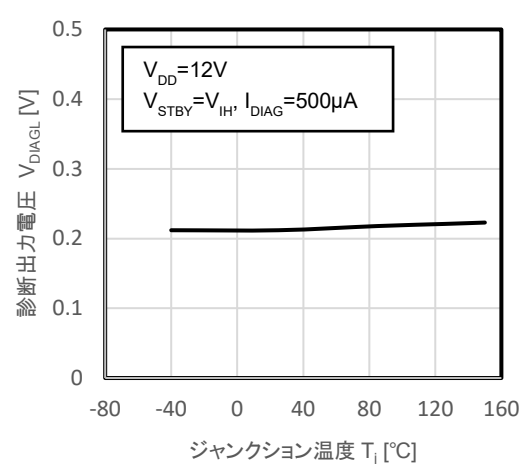
図 12.22 V_{DIAGL} - T_j
