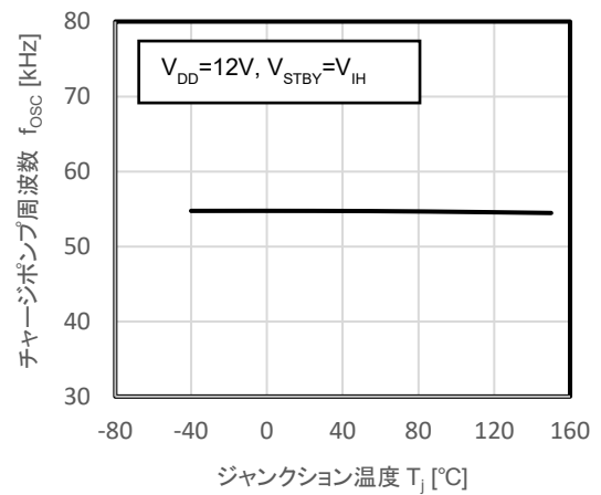
図 12.24 f_{osc} - T_j
