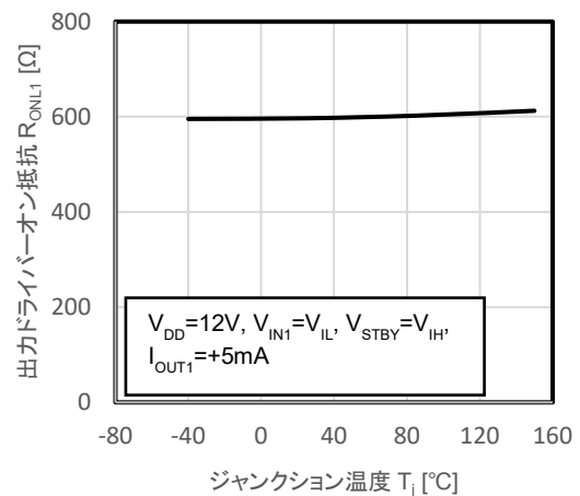
図 12.32 R_{ONL1} - T_j
