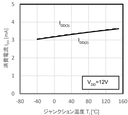
図 12.3 I_{DD} - T_j
