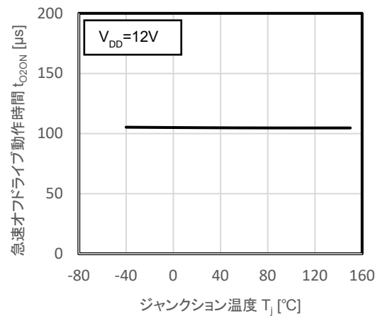
図 12.38 t_{O2ON} - T_j
