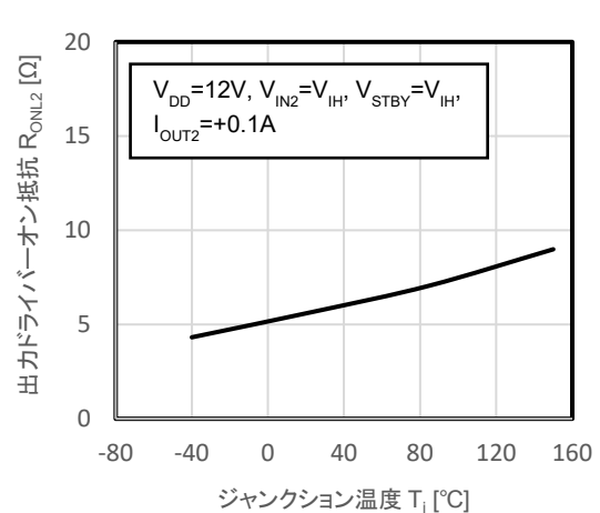
図 12.34 R_{ONL2} - T_j
