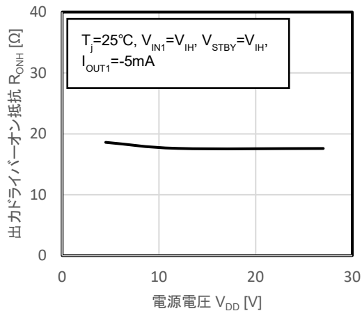
図 12.29 R_{ONH} - V_{DD}
