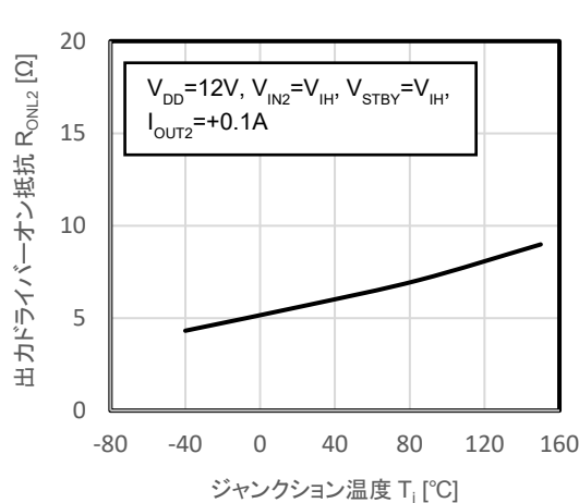
図 12.34 R_{ONL2} - T_j
