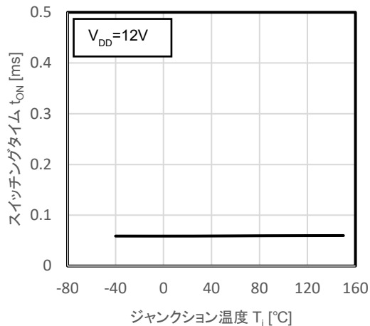
図 12.35 t_{ON} - T_j
