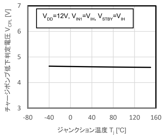
図 12.26 V_{CPL} - T_j
