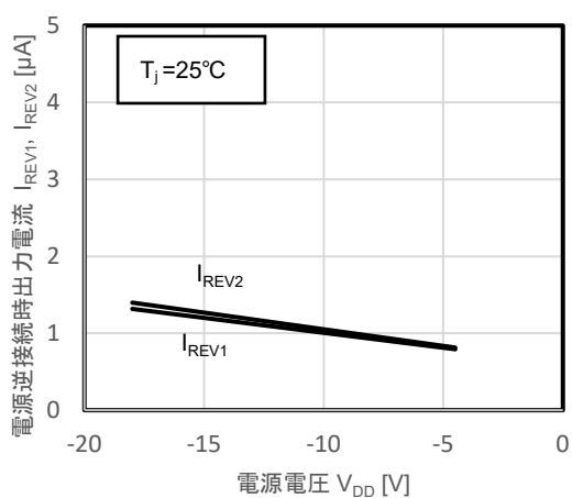
図 12.39 I_{REV1} , I_{REV2} - V_{DD}
