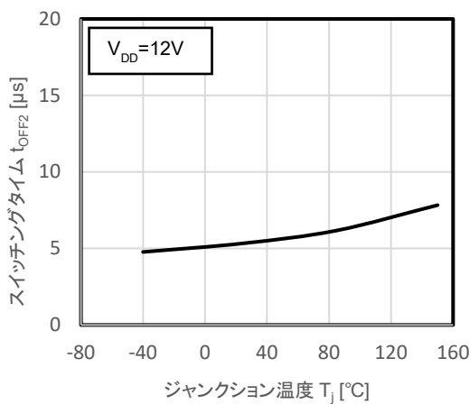
図 12.37 t_{OFF2} - T_j
