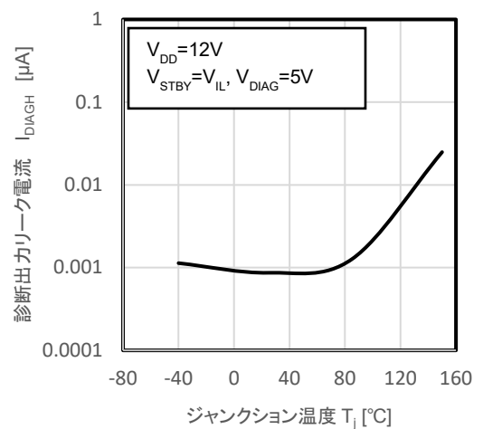
図 12.20 I_{DIAGH} - T_j
