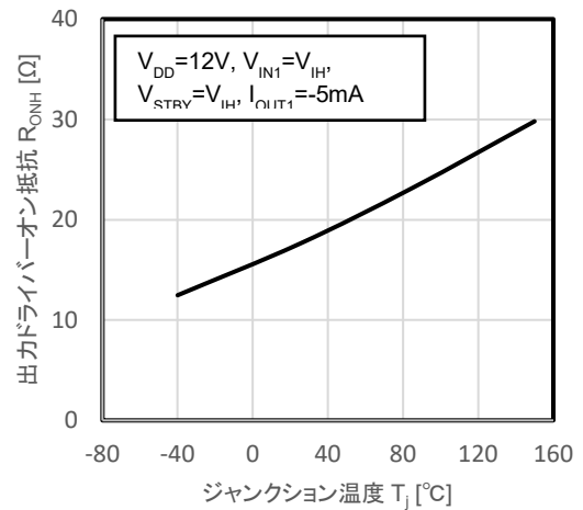
図 12.30 R_{ONH} - T_j
