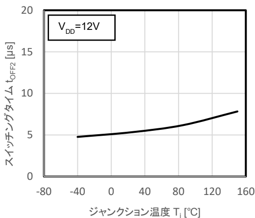
図 12.37 t_{OFF2} - T_j
