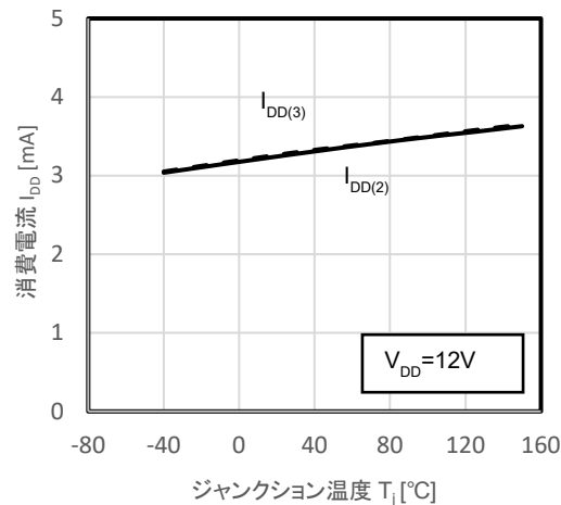
図 12.3 I_{DD} - T_j
