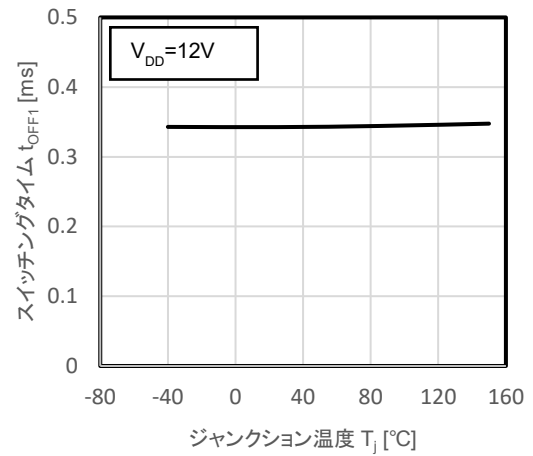
図 12.36 t_{OFF1} - T_j
