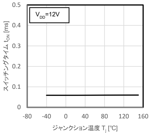
図 12.35 t_{ON} - T_j
