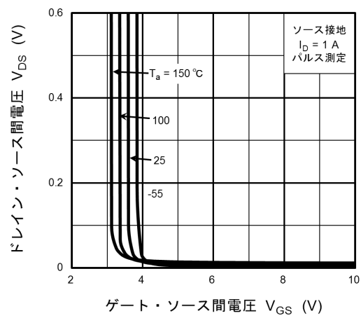
図 8.6 V_{DS} - V_{GS}
