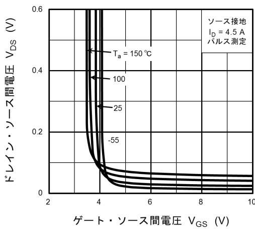
図 8.5 V_{DS} - V_{GS}
