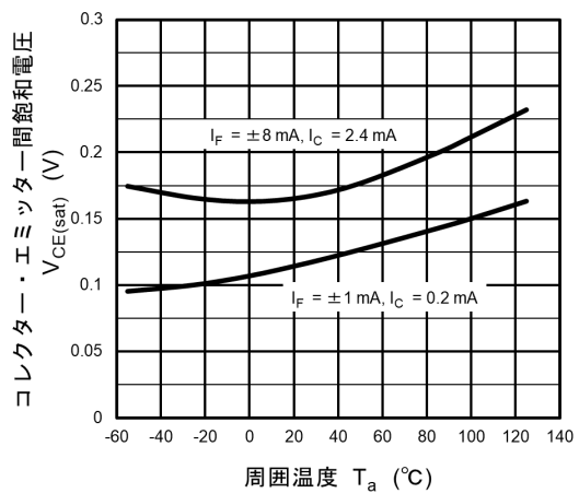
図 12.10 V_{CE(sat)} - T_a
