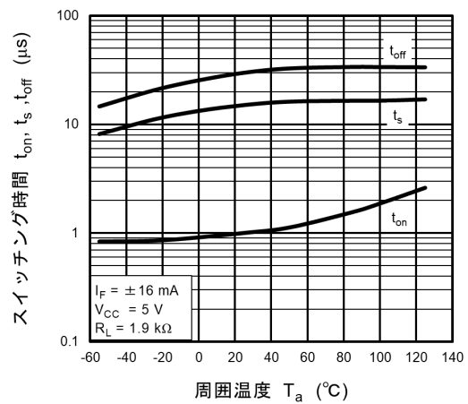
図 12.16 スwitchング時間 - T_a
