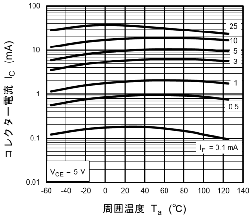
図 12.13 I_C - T_a
