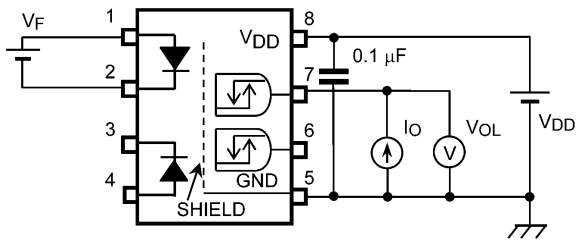
図 12.1.1 VOL測定回路
