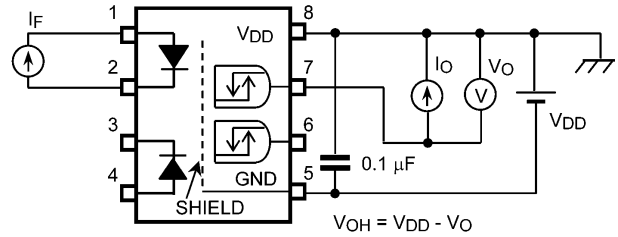
図 12.1.2 VOH測定回路
