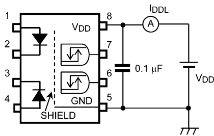
図 12.1.3 IDD L測定回路
