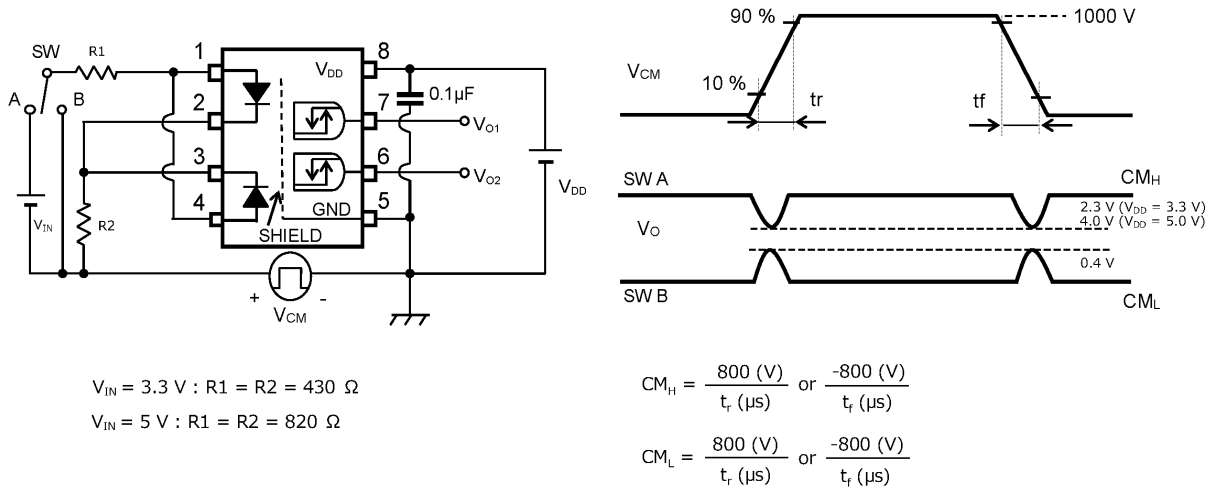
図 12.1.7 コモンモード過渡耐性測定回路, 波形
