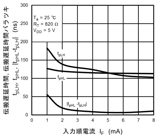
図 12.2.14 t_{pLH} , t_{pHL} , |t_{pHL} - t_{pLH}| - I_F
