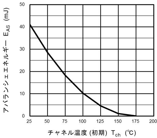
図 8.15 E_{AS} - T_{ch}
