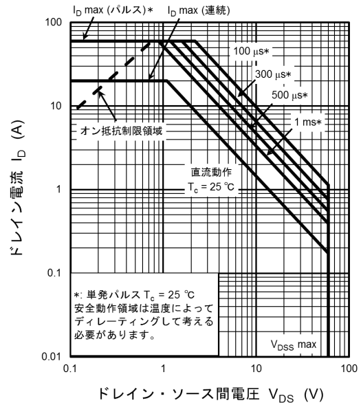
図 8.19 安全動作領域 (最大値 (保証値))
