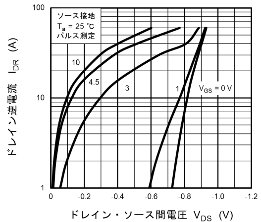
図 8.10 I_{DR} - V_{DS}
