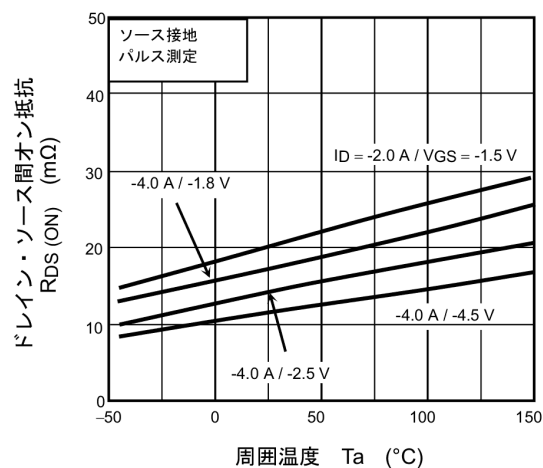
図 8.6 R_{DS(ON)} - T_a
