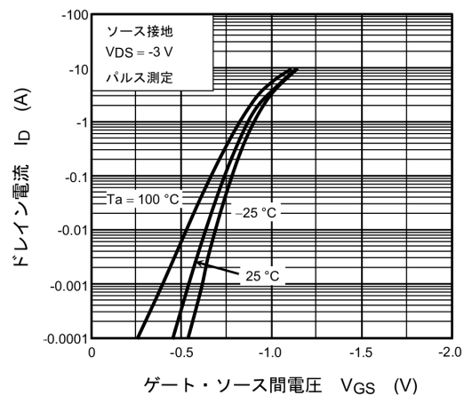
図 8.2 I_D - V_{GS}
