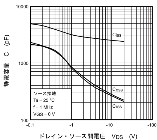
図 8.9 C - V_{DS}
