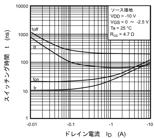
図 8.11 t - I_D
