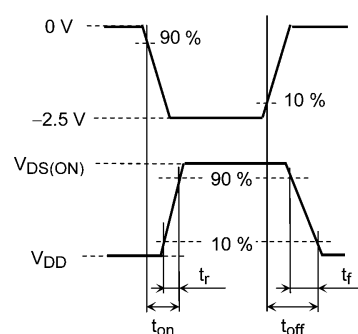
図 6.3.2 入力波形/出力波形
