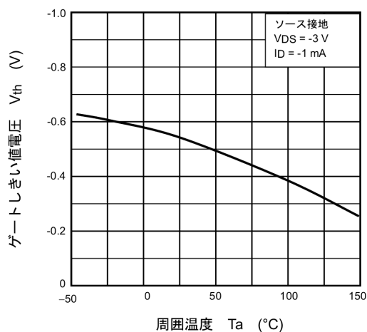
図 8.7 V_{th} - T_a
