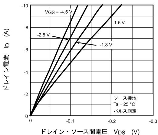
図 8.1 I_D - V_{DS}
