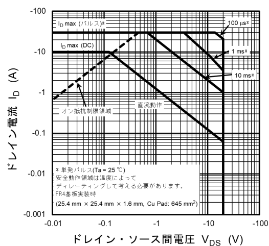
図 8.15 安全動作領域
