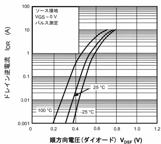
図 8.12 I_{DR} - V_{DSF}
