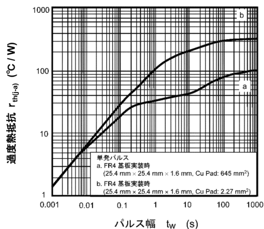
図 8.13 r_{th(j-a)} - t_w
