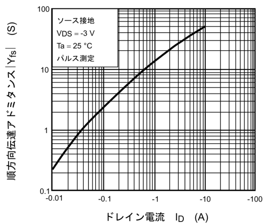
図 8.8 |Y_{fs}| - I_D
