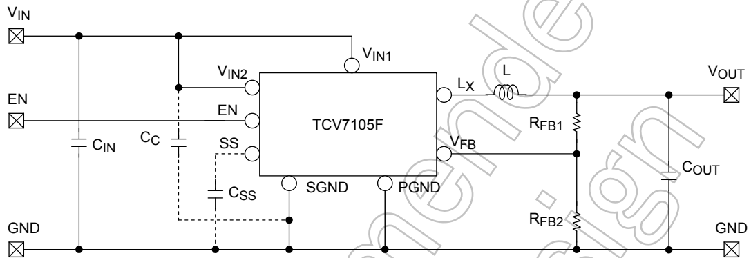
図 1 TCV7105F 応用回路例
