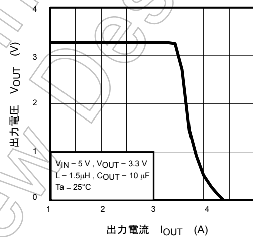
過電流特性
