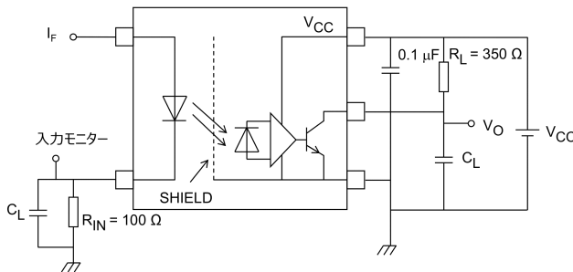
図 12.1.5 伝搬遅延時間測定回路, 波形
