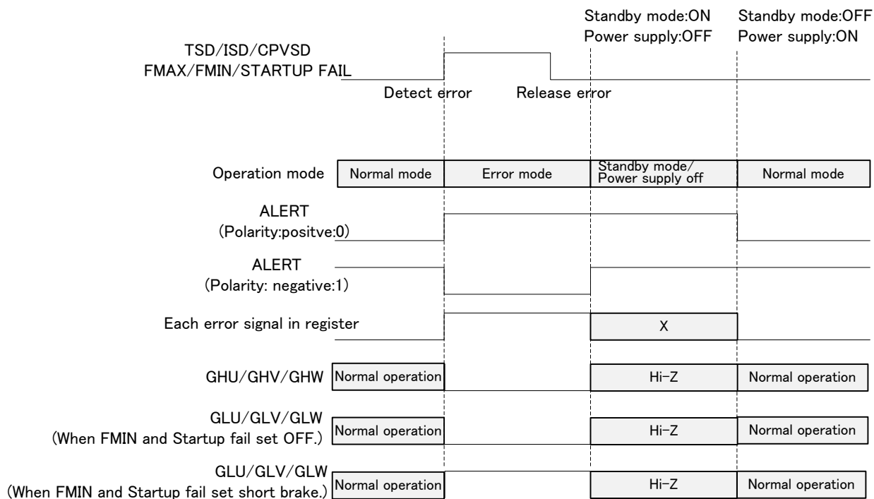
図 8.25 ラッチ方式時エラーモードのスタンバイモード/電源 OFF 解除のタイミングチャート例
