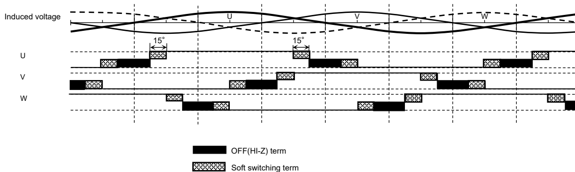
図 8.5 通電波形のタイミングチャート
