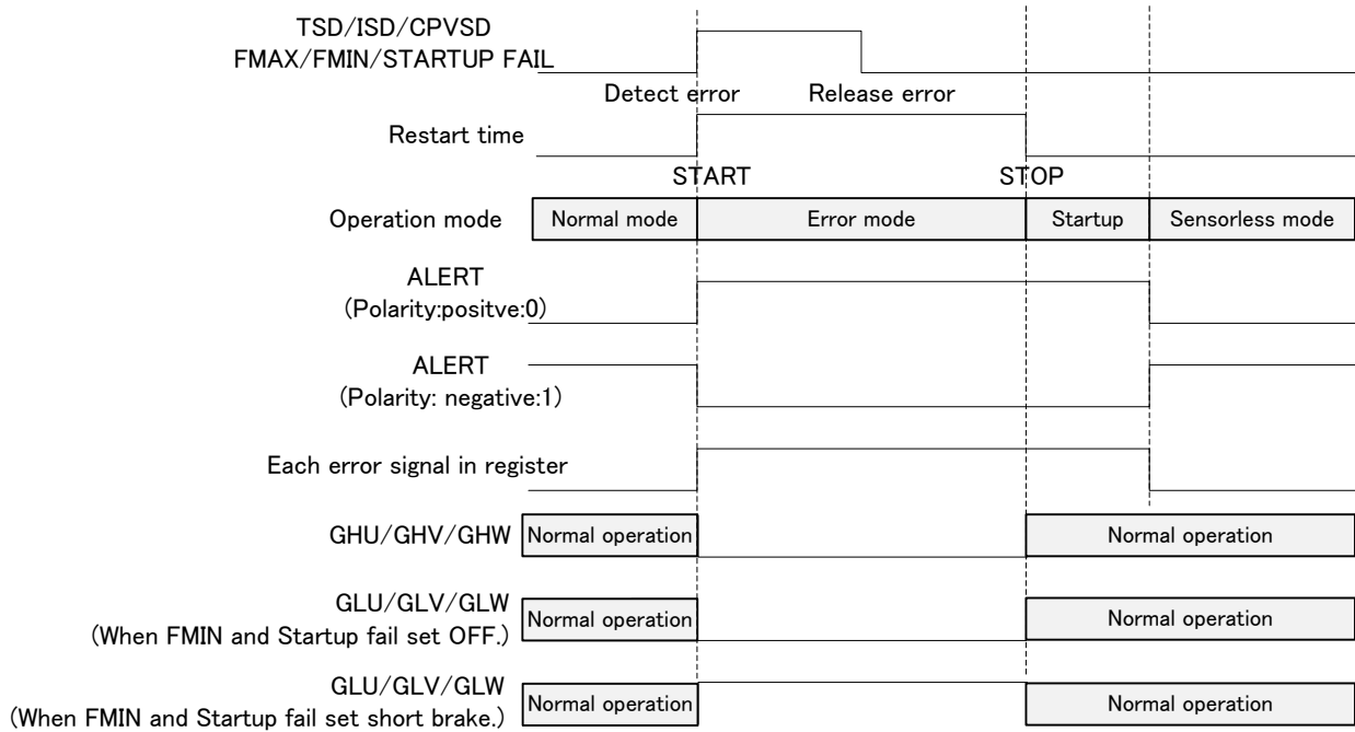
図 8.23 自動復帰方式時のエラーモードのタイミングチャート例
