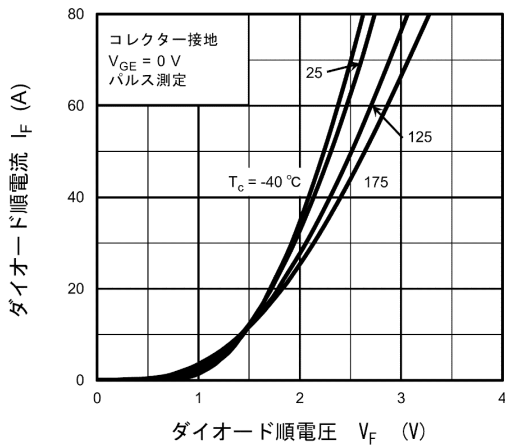
ダイオード順電圧 V_F (V) 図 8.11 I_F - V_F
