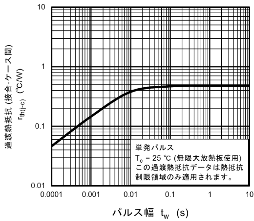
パルス幅 t_w (s) 図 8.9 r_{th(j-c)} - t_w (最大値 (保証値))
