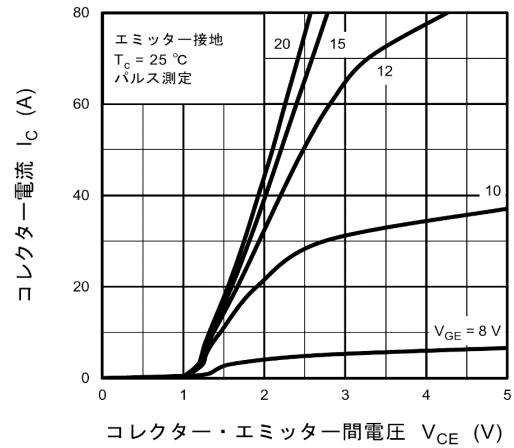
図 8.2 I_C - V_{CE}
