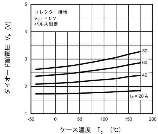
ケース温度 T_c (°C) 図 8.12 V_F - T_c
