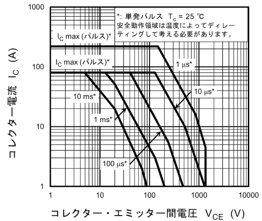
コレクター・エミッター間電圧 V_{CE} (V) 図 8.10 安全動作領域 (最大値 (保証値))
