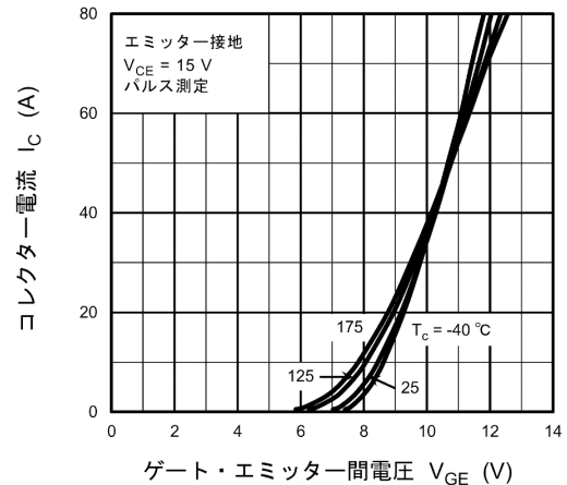
図 8.6 I_C - V_{GE}
