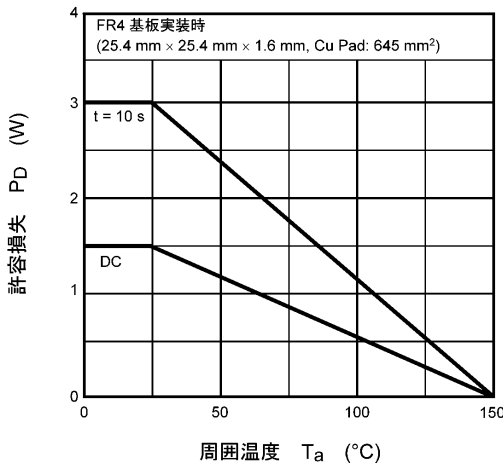
図 7.11 P_D - T_a
