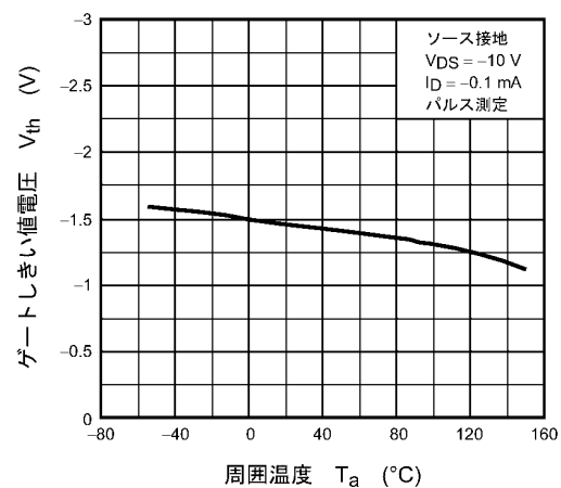
図 7.6 V_{th} - T_a
