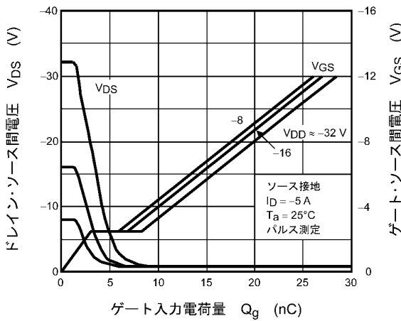
図 7.9 ダイナミック入力特性
