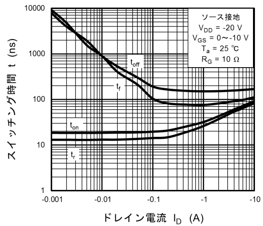
図 7.10 t - I_D
