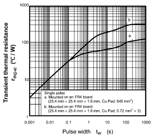
Fig. 8.11 r_{th(j-a)} - t_w
