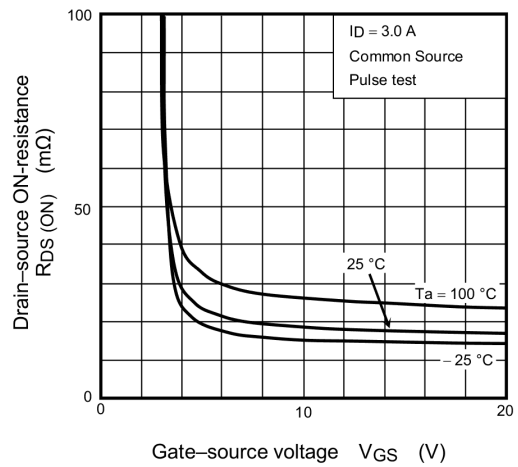
Fig. 8.3 R_{DS(ON)} - V_{GS}
