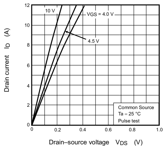
Fig. 8.1 I_D - V_{DS}
