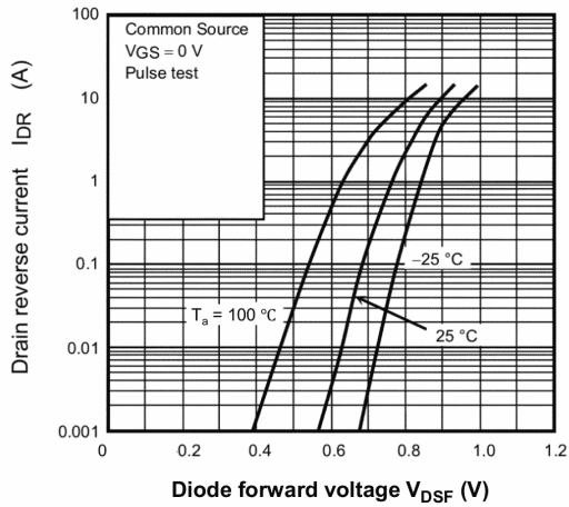
Fig. 8.7 I_{DR} - V_{DSF}
