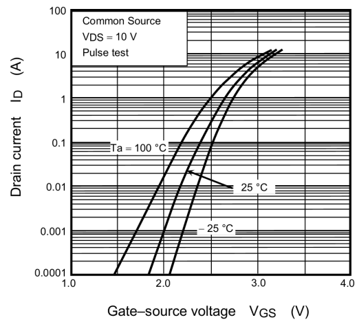
Fig. 8.2 I_D - V_{GS}
