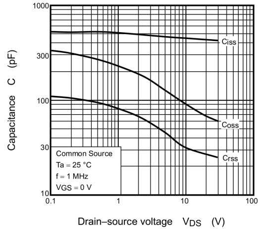
Fig. 8.8 C - V_{DS}
