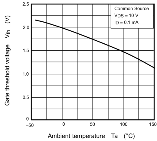
Fig. 8.6 V_{th} - T_a
