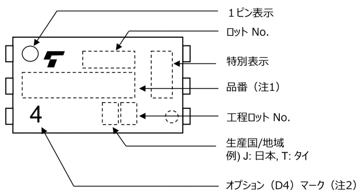
図 17.3 現品表示例
