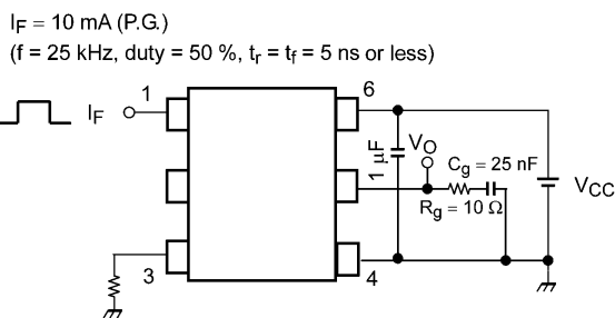
图 13.1.7 伝搬遅延時間測定回路, 波形
