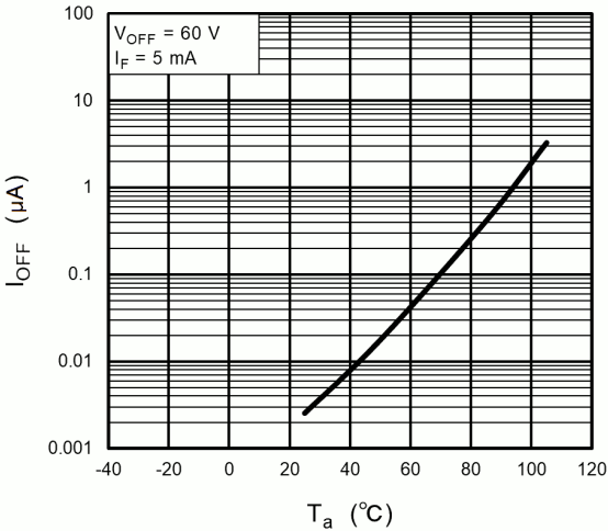
Fig. 12.8 I_{OFF} - T_a
