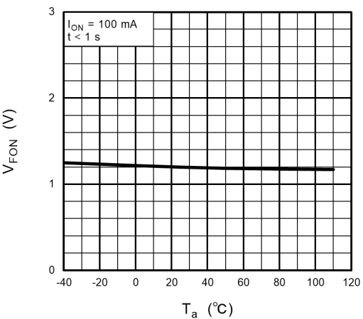
Fig. 12.4 V_{FON} - T_a
