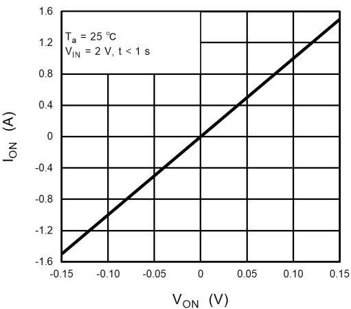
Fig. 12.2 I_{ON} - V_{ON}
