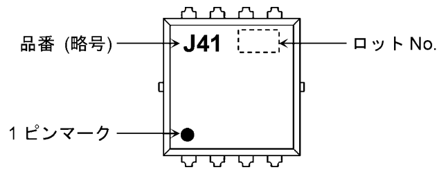
図 7.1 現品表示
